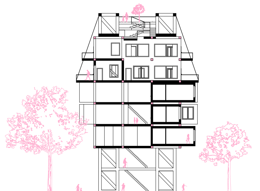
Schnitt 1:400
