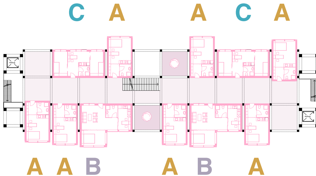
Grundriss 4.OG 1:400
