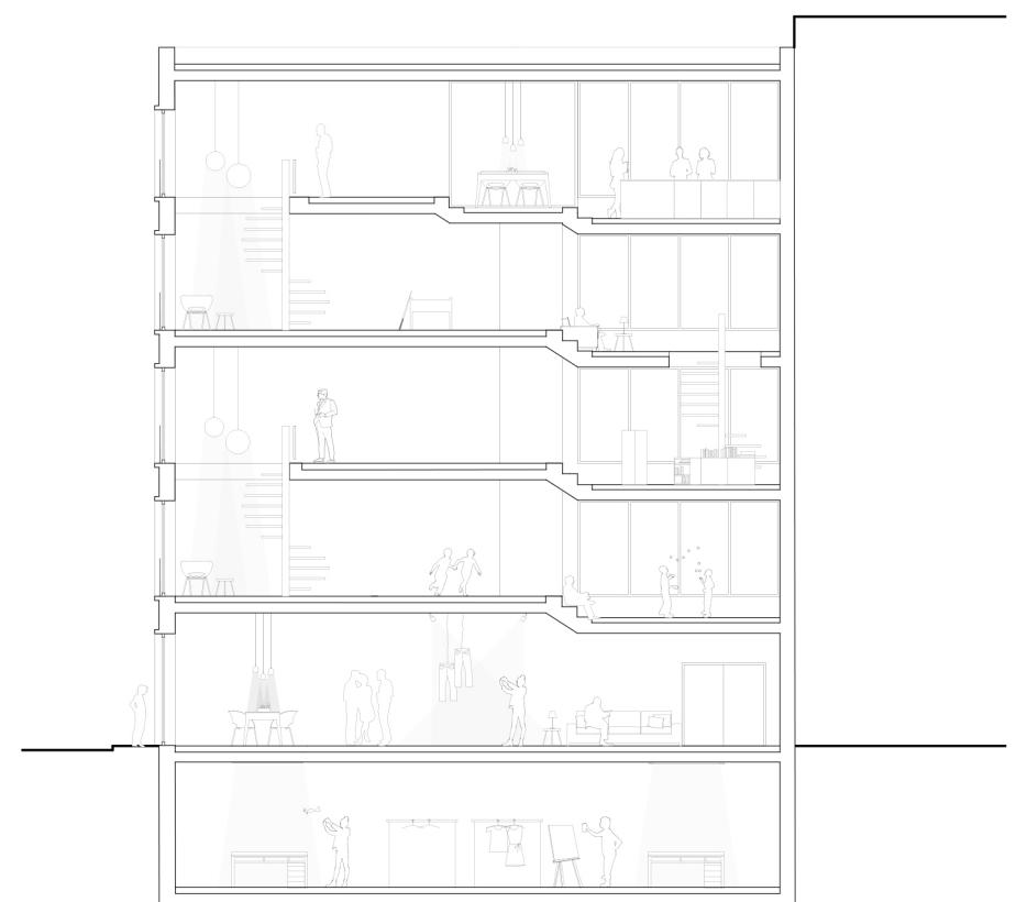
Schnitt C-C | 1:200
