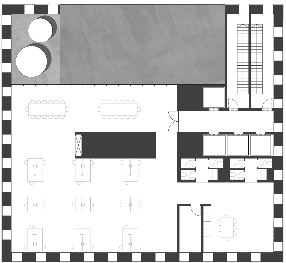
Grundriss 7.OG 1:200
