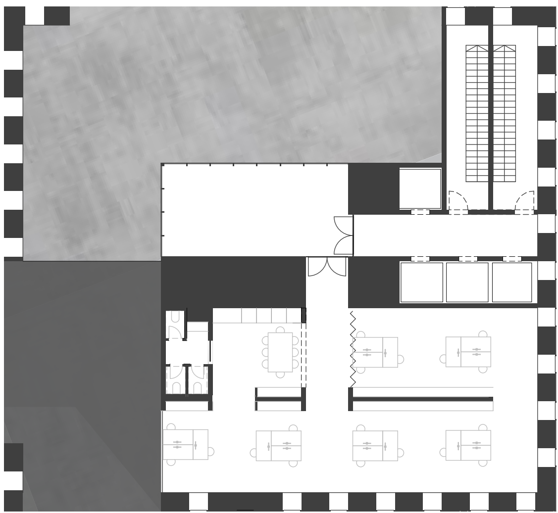
Grundriss 4.OG 1:200
