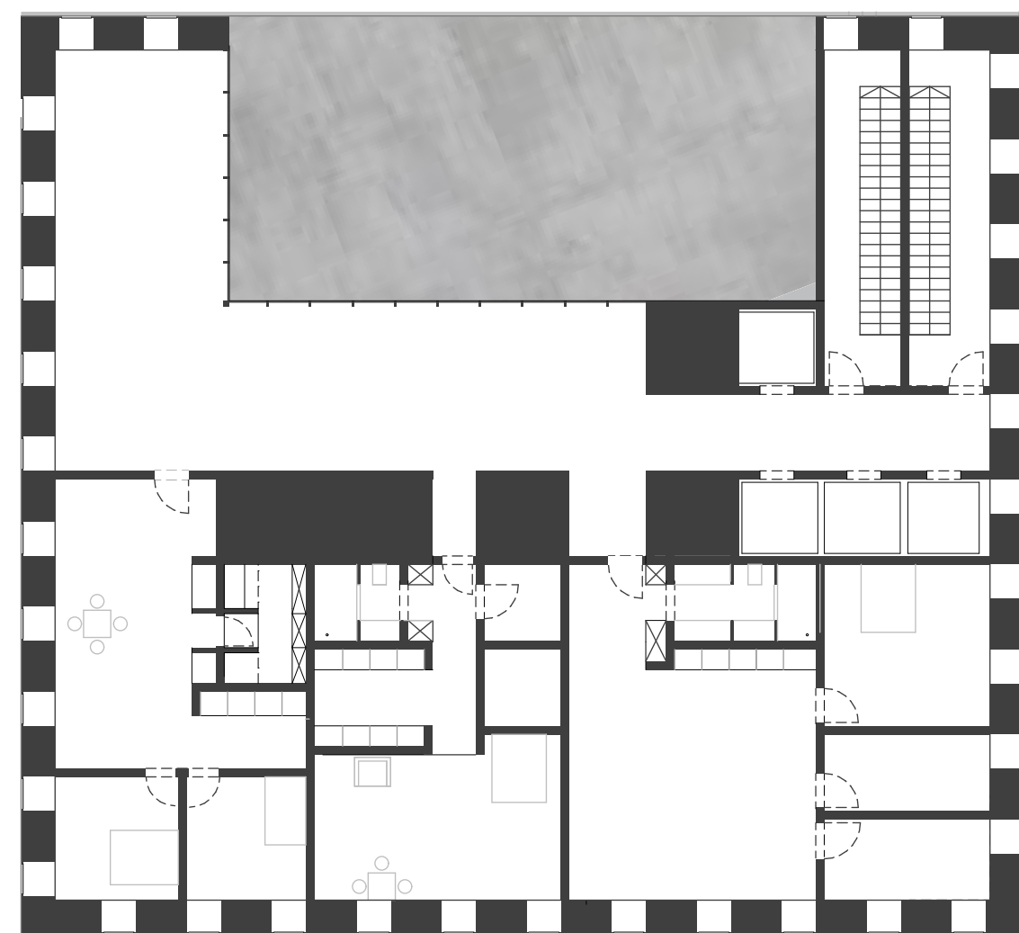
Grundriss 6.OG 1:200
