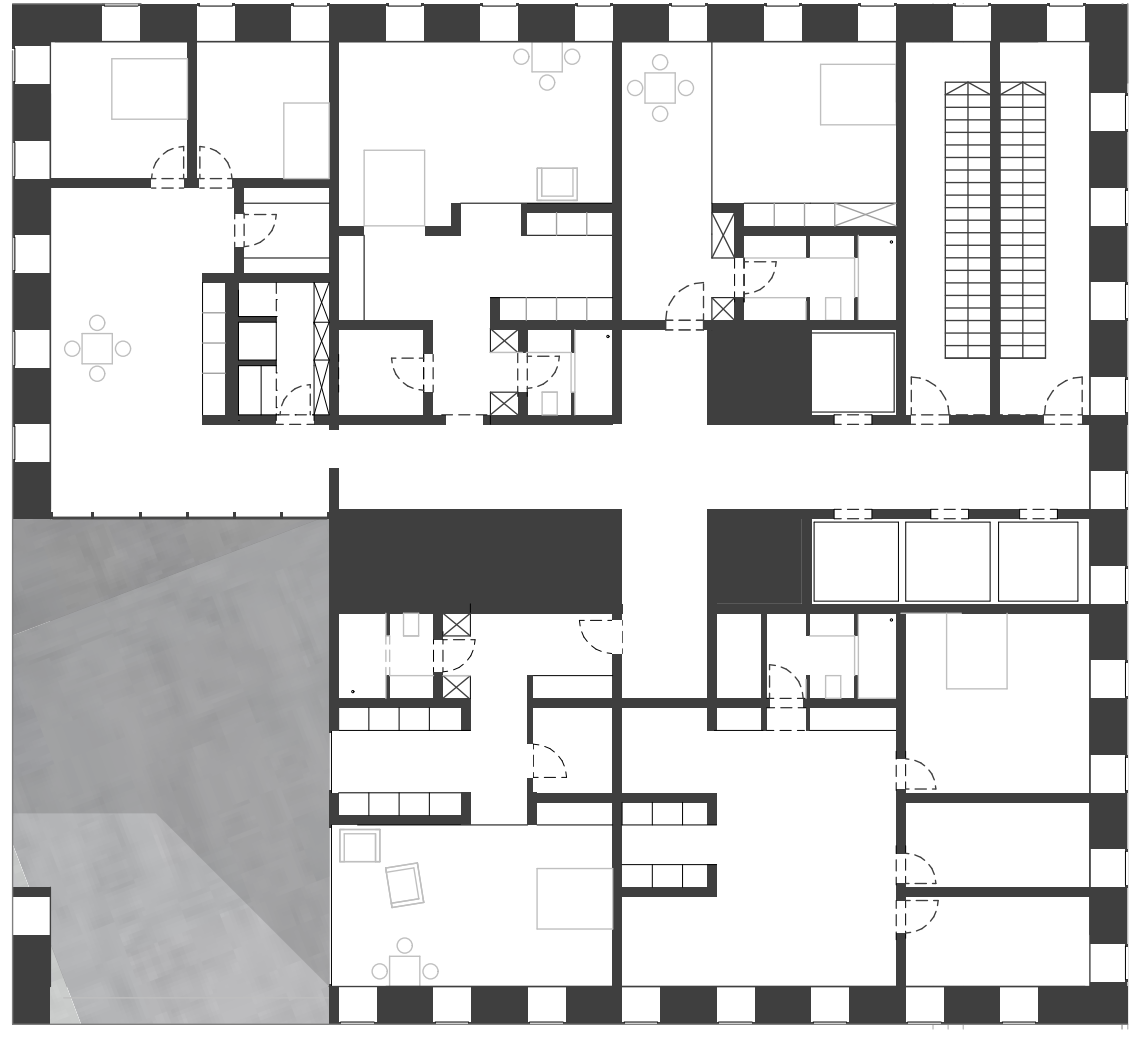
Grundriss 3.OG 1:200
