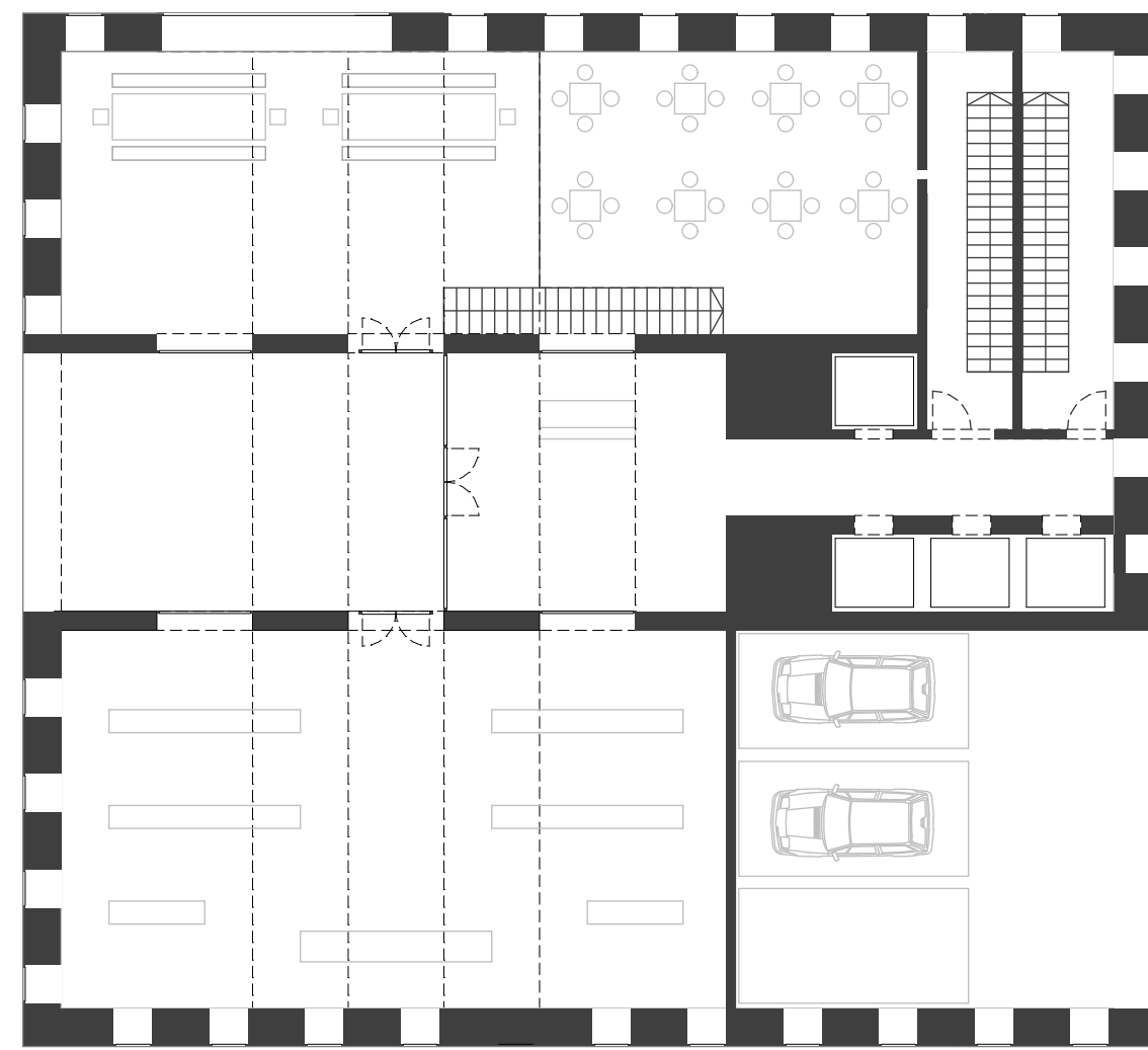
Grundriss EG 1:200
