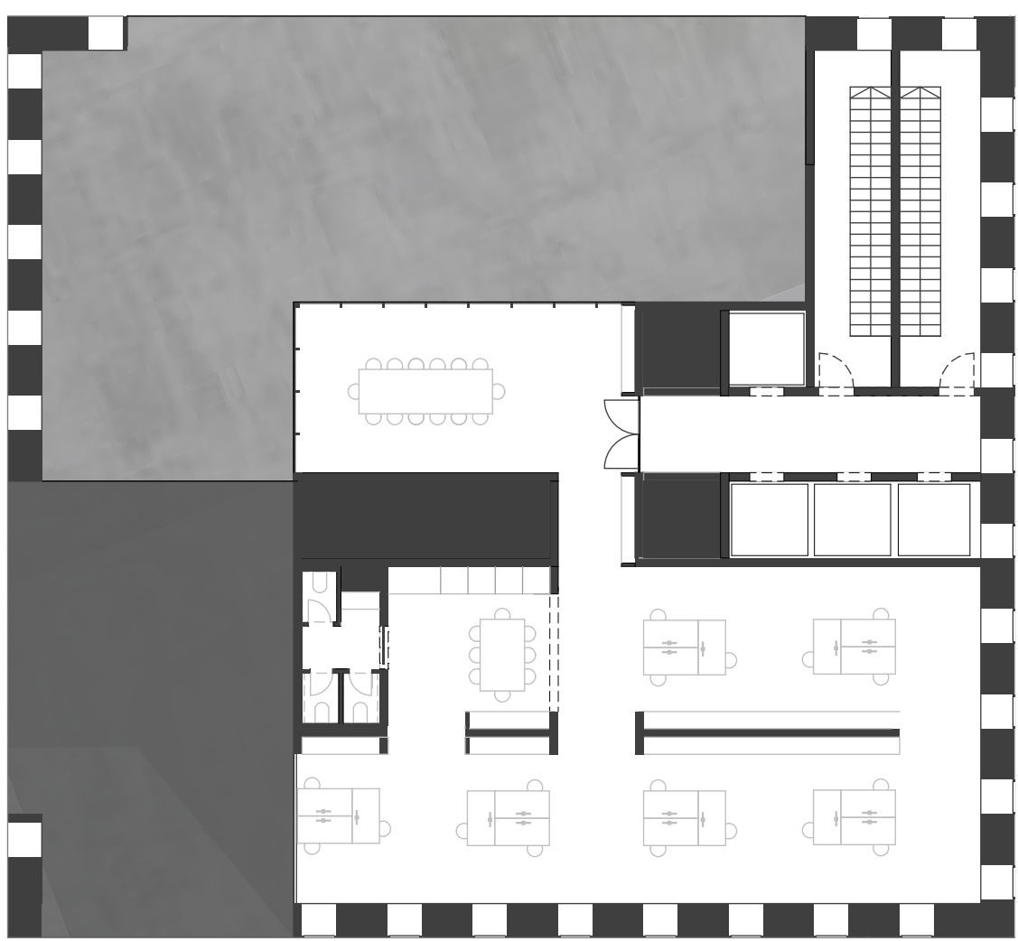
Grundriss 5.OG 1:200
