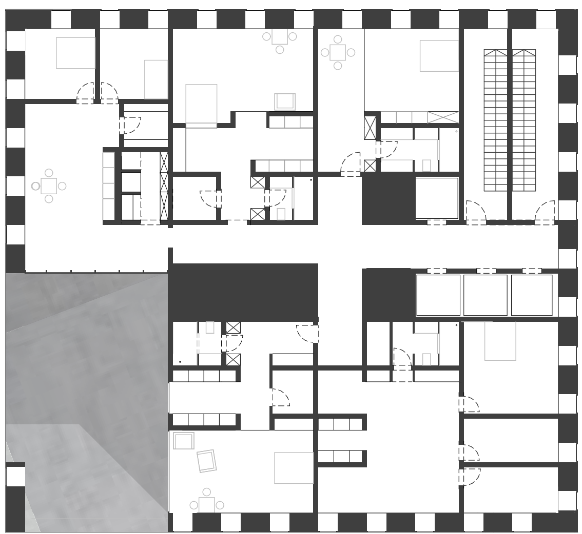
Grundriss 1.OG 1:200
