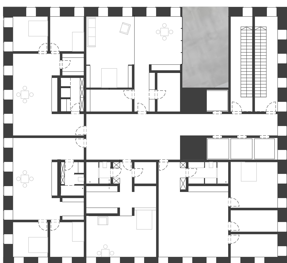
Grundriss 11.OG 1:200
