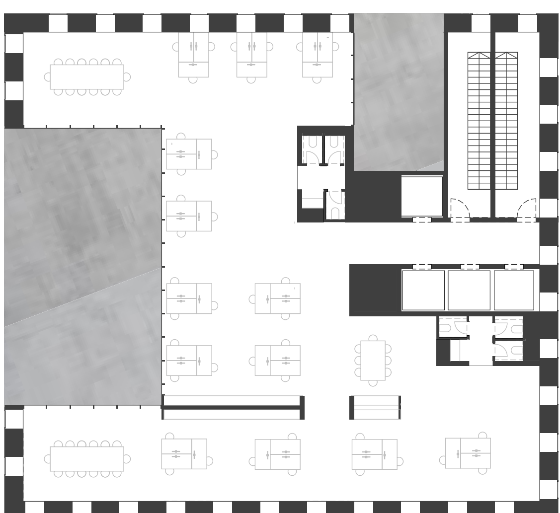
Grundriss 13.OG 1:200
