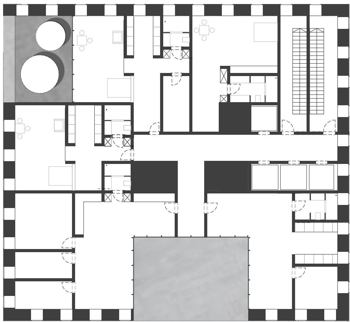
Grundriss 8.OG 1:200
