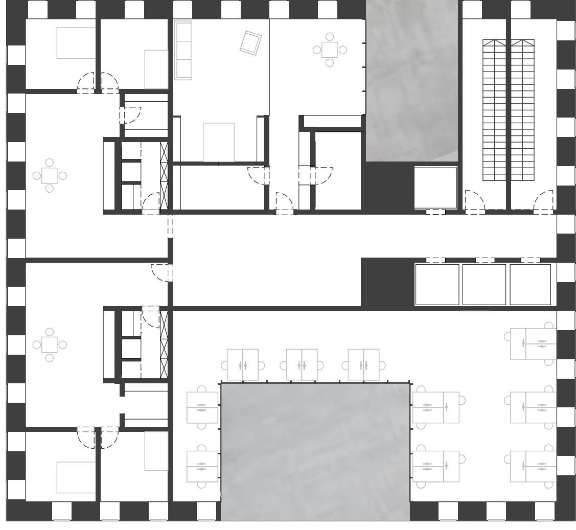
Grundriss 10.OG 1:200
