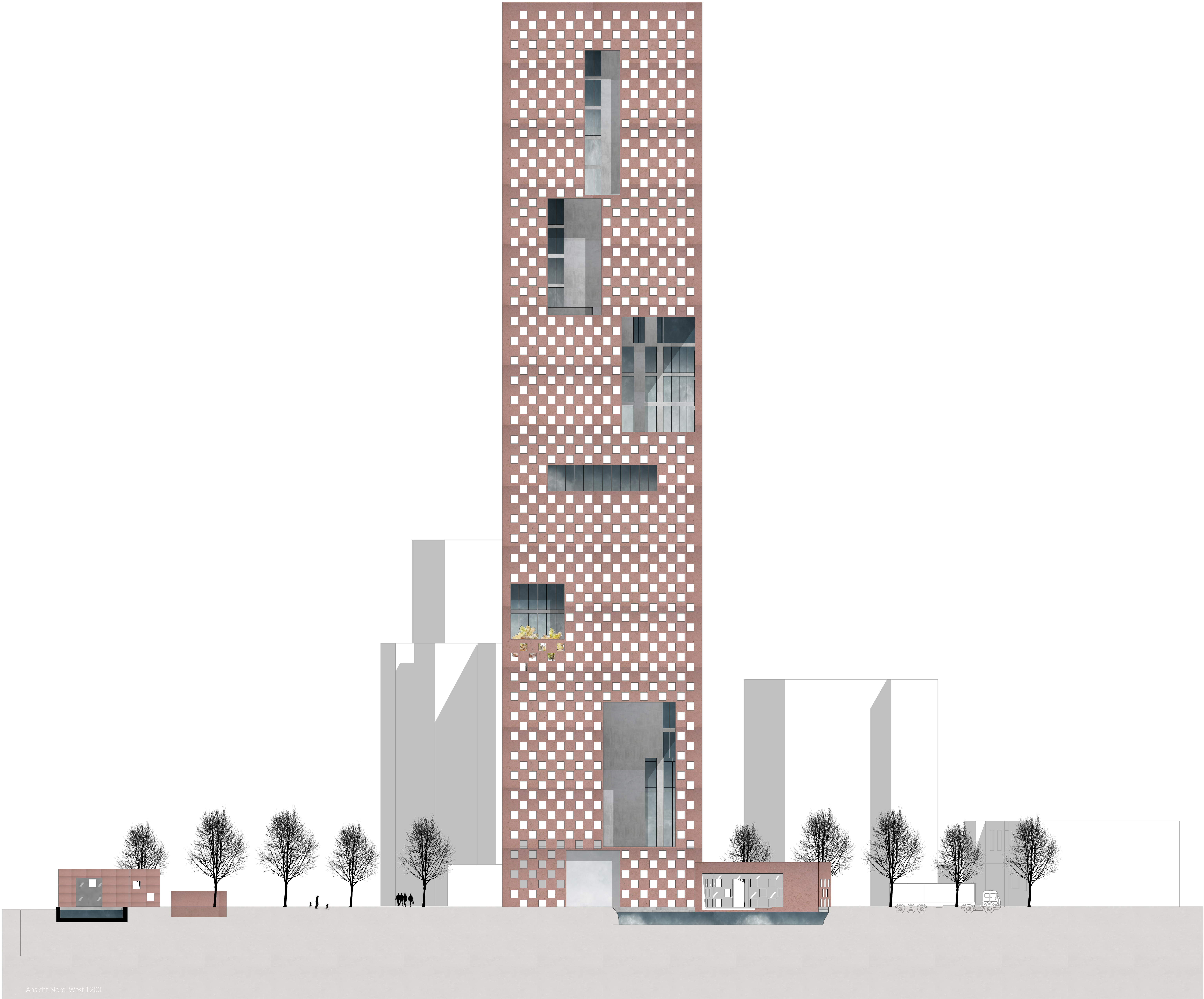
Ansicht Nord-West 1:200
