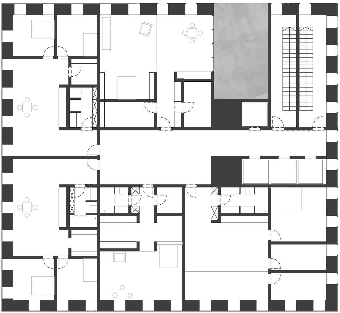
Grundriss 14.OG 1:200
