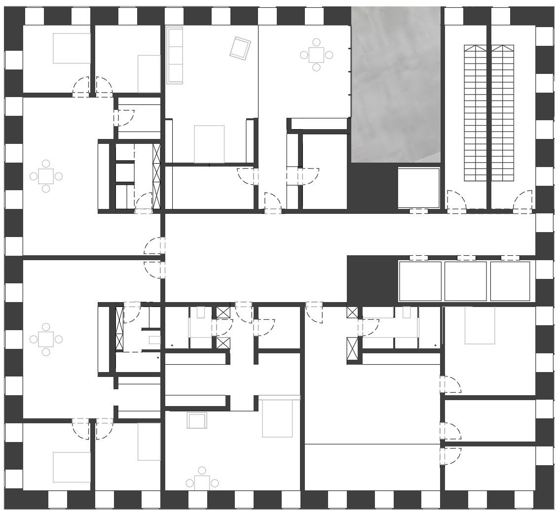
Grundriss 12.OG 1:200
