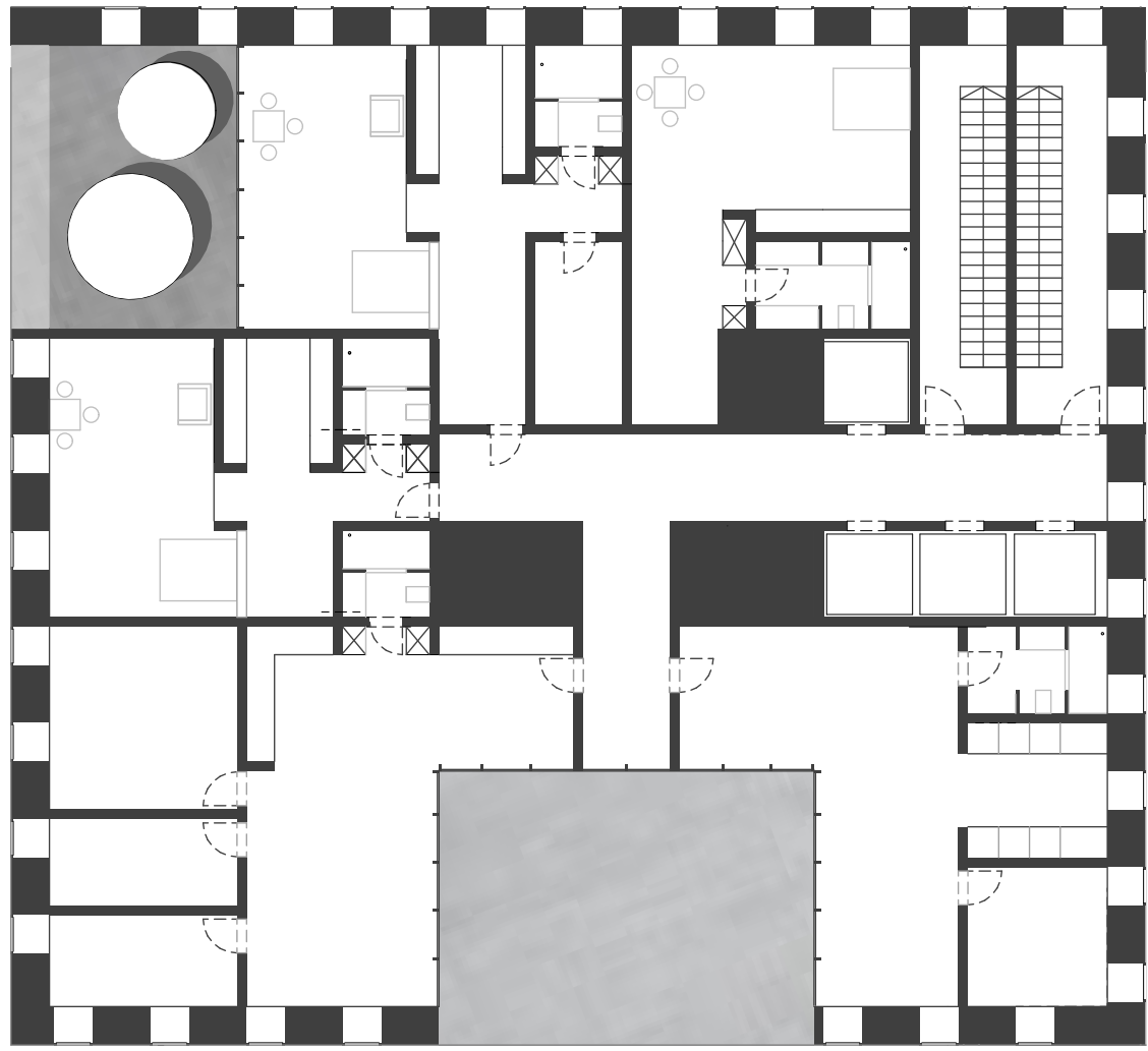
Grundriss 9.OG 1:200
