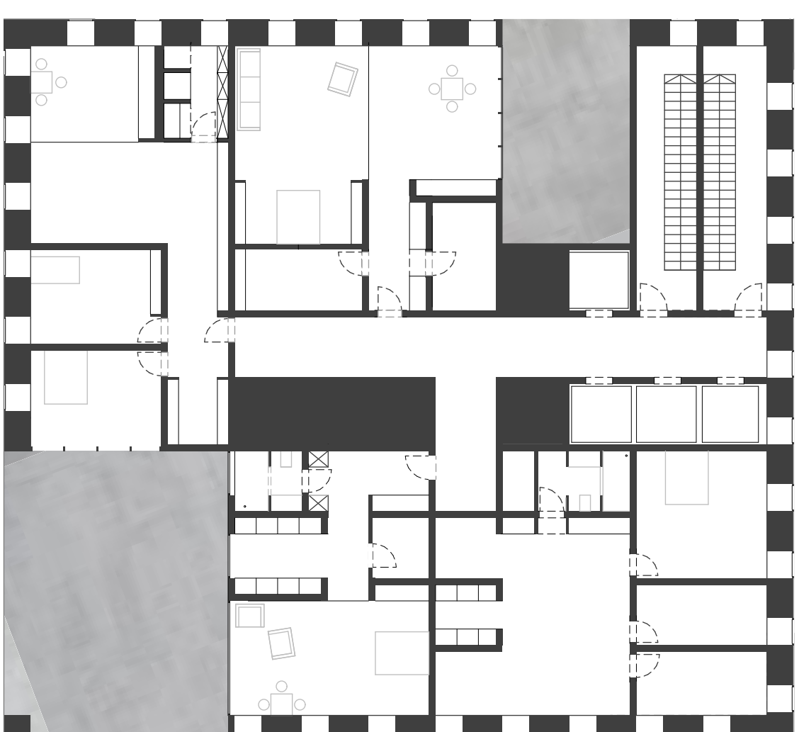
Grundriss 15.OG 1:200
