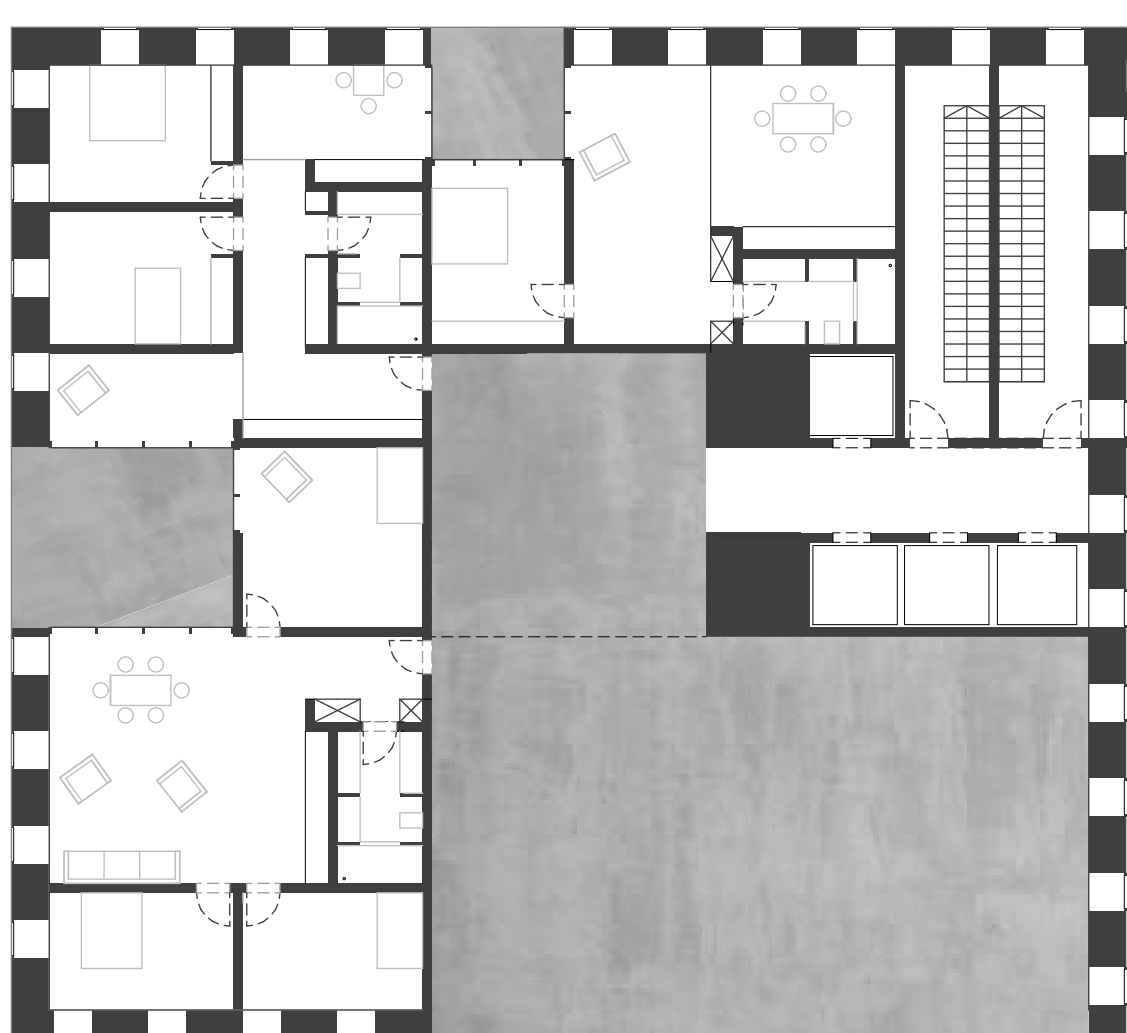
Grundriss 23.OG 1:200
