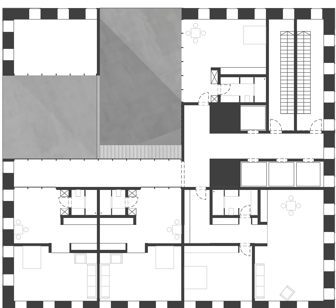
Grundriss 21.OG 1:200
