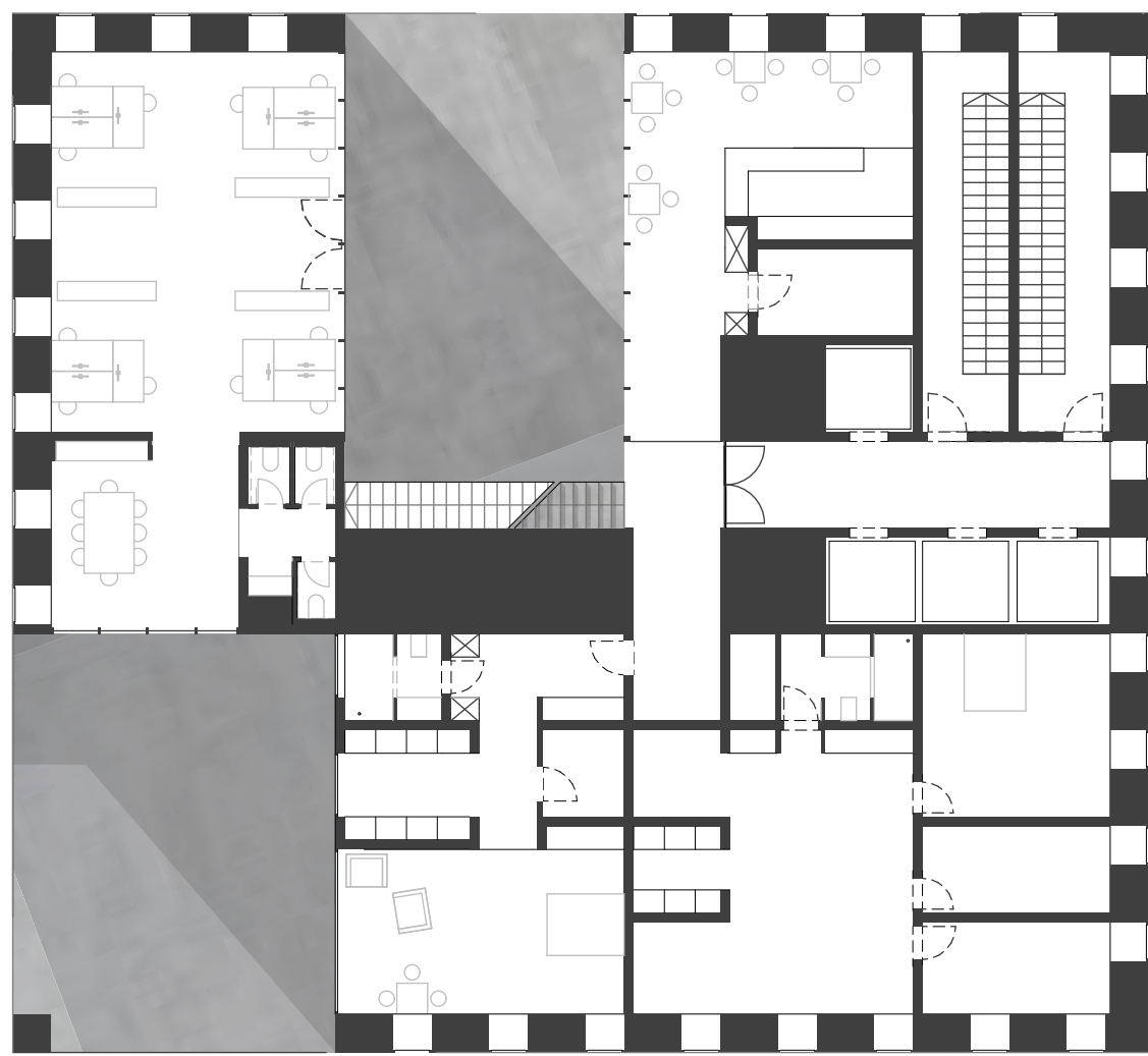
Grundriss 18.OG 1:200
