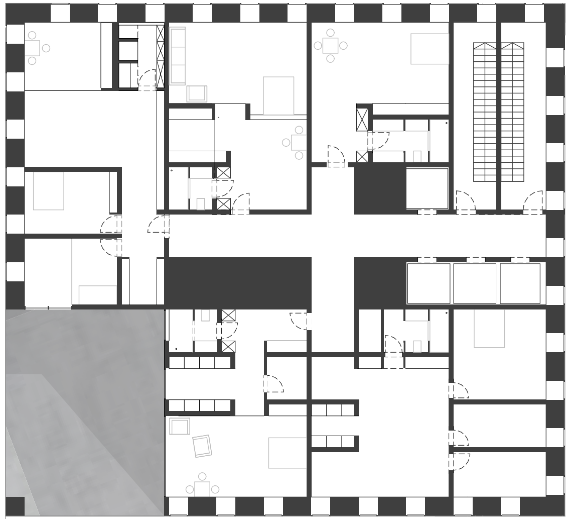
Grundriss 17.OG 1:200
