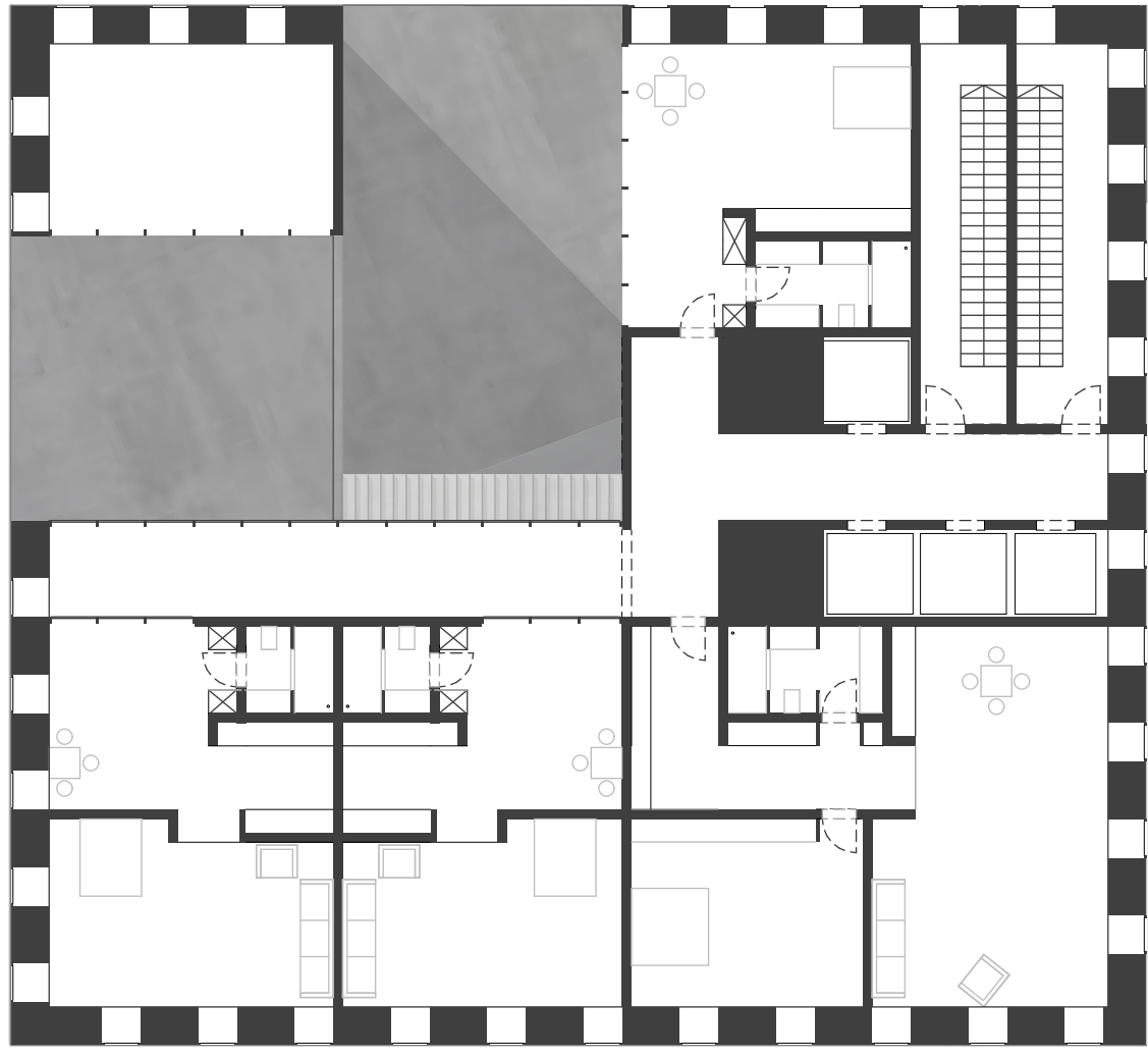
Grundriss 20.OG 1:200
