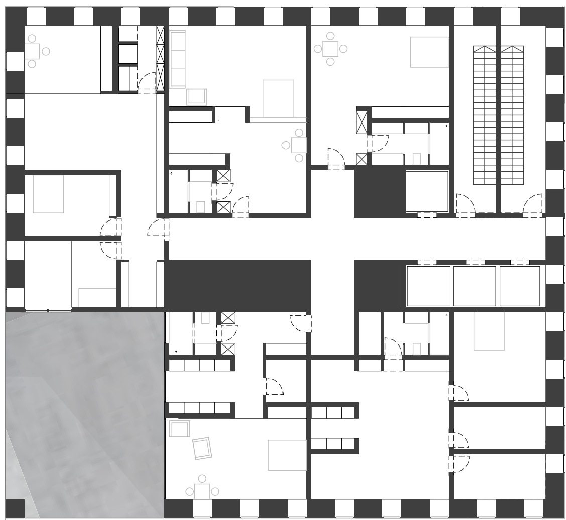
Grundriss 16.OG 1:200
