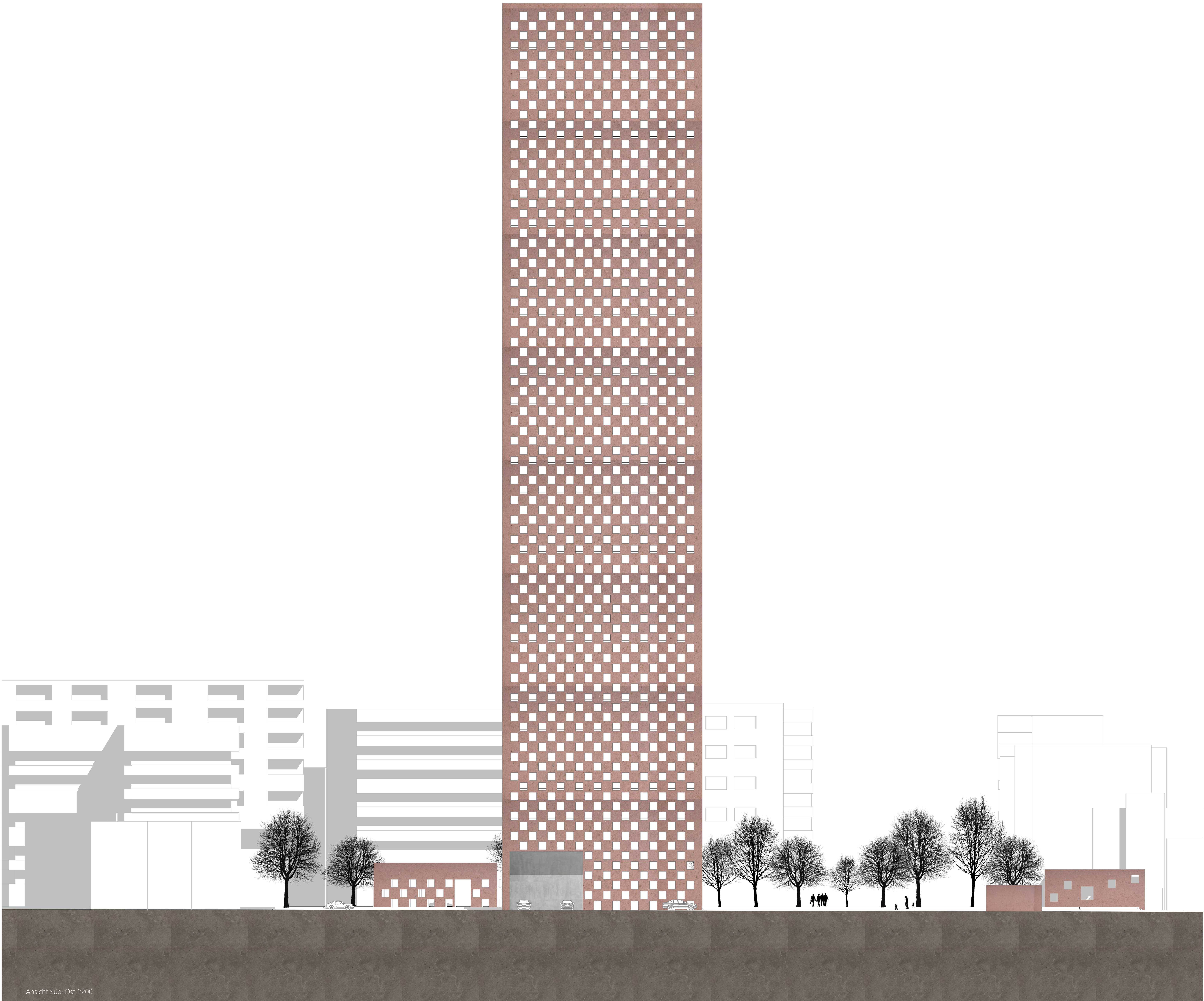
Ansicht Süd-Ost 1:200
