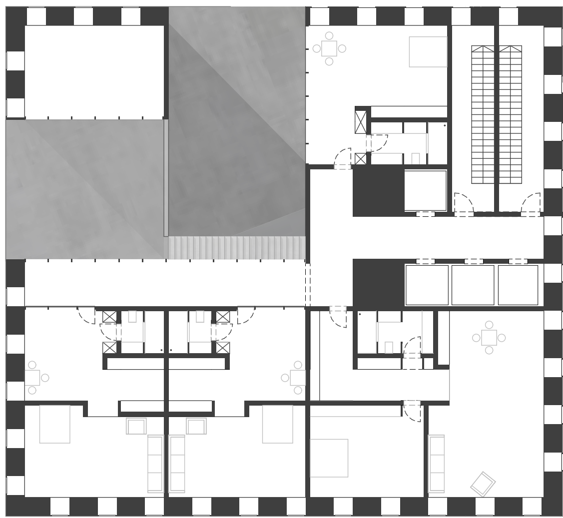
Grundriss 22.OG 1:200
