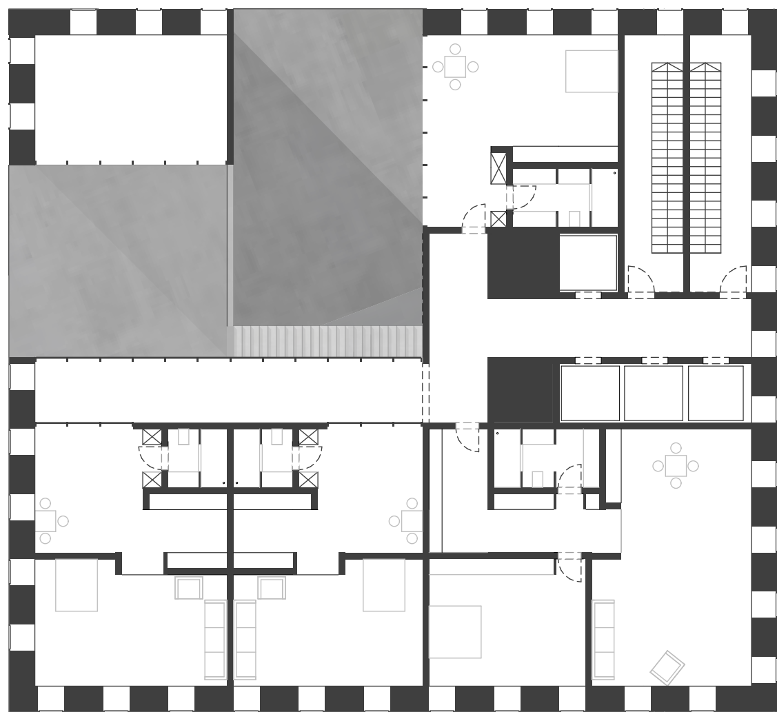
Grundriss 19.OG 1:200
