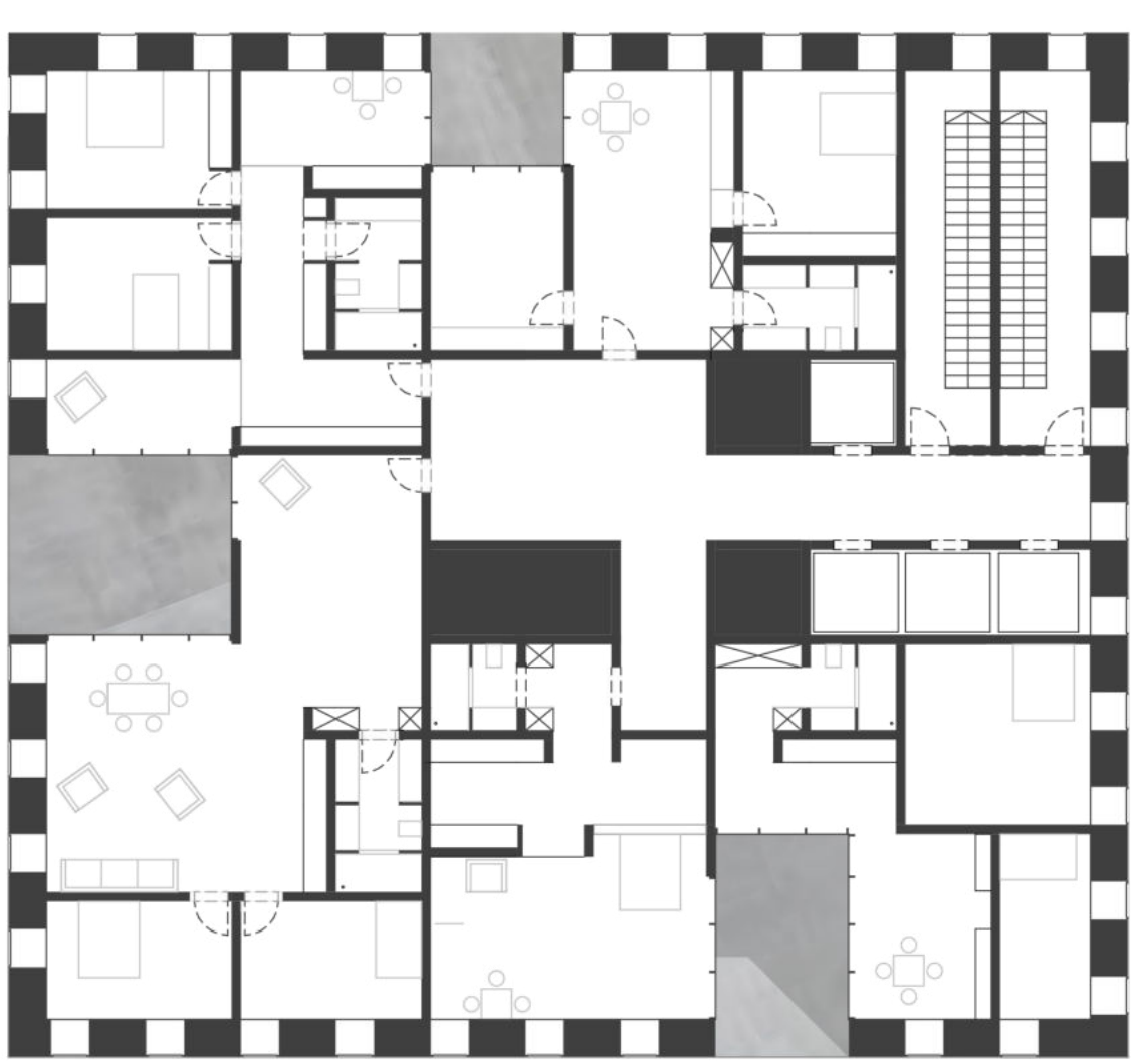
Grundriss 25.OG 1:200
