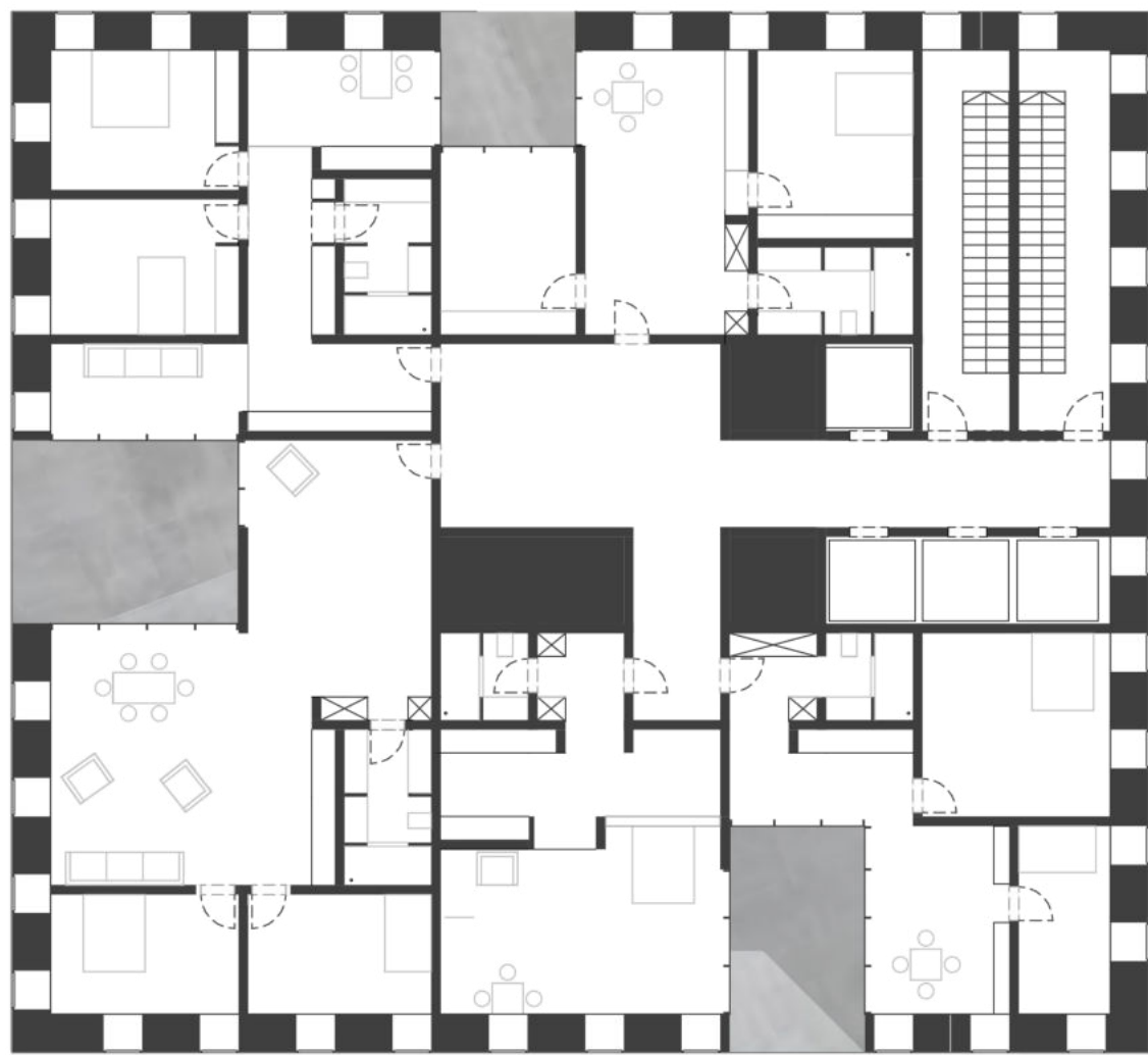
Grundriss 26.OG 1:200
