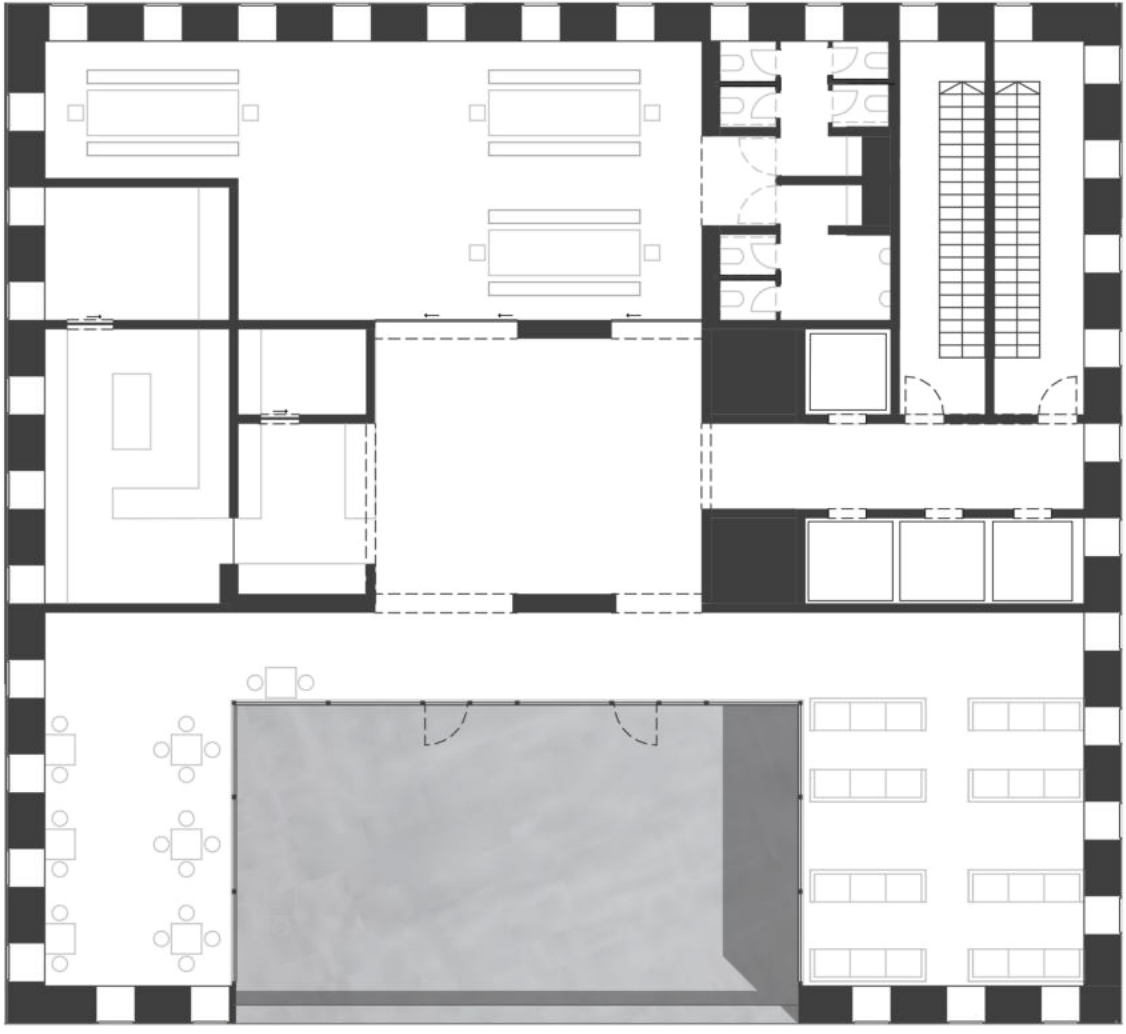
Grundriss 28.OG 1:200
