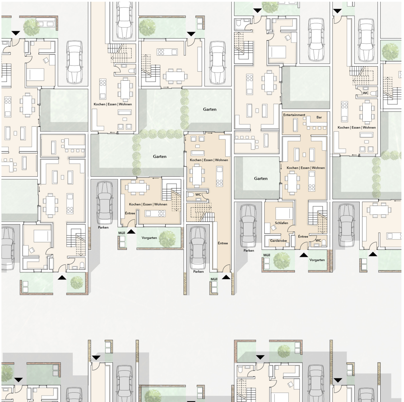
grundriss erdgeschoss m 1:100
