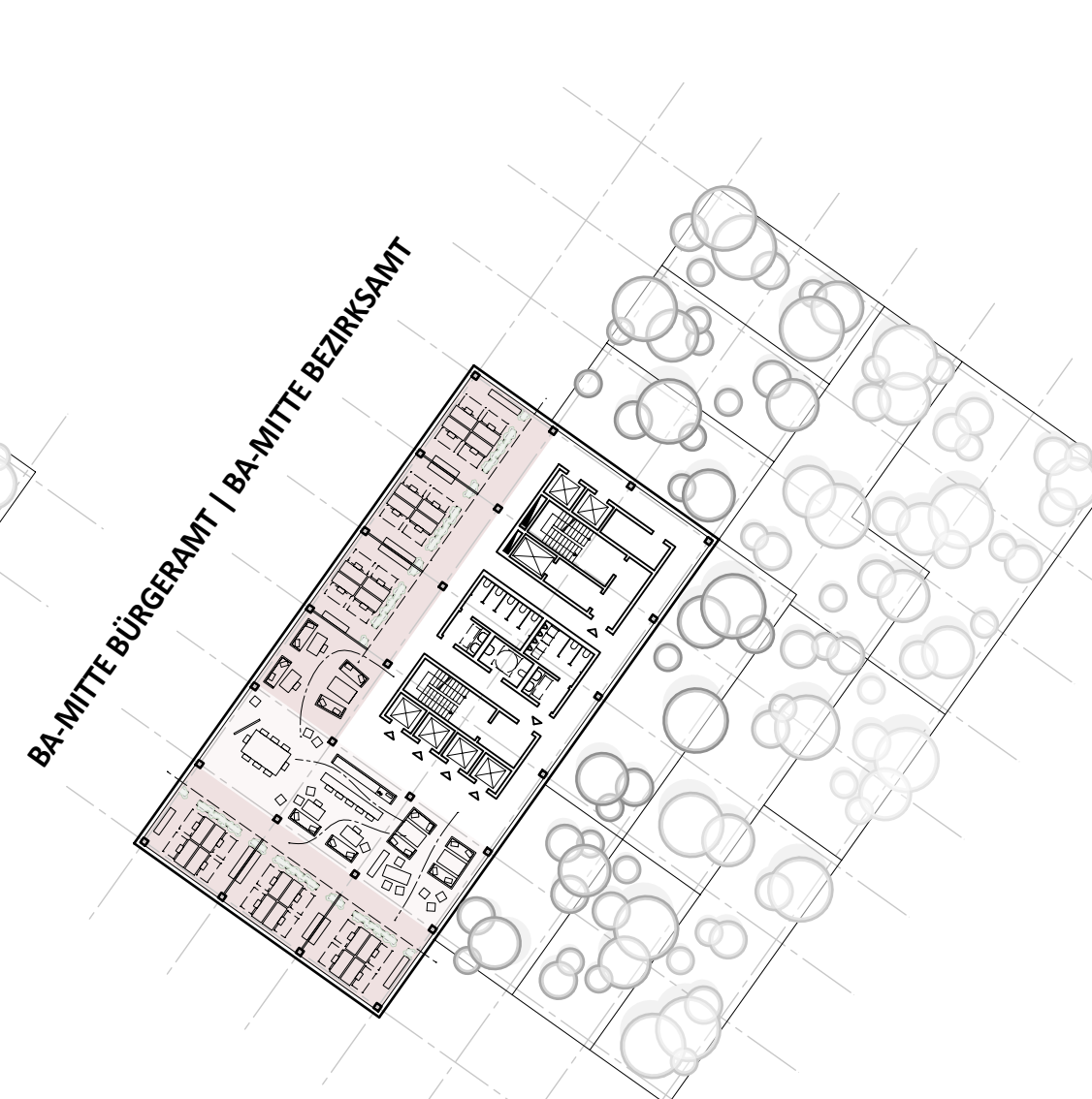
Grundriss | 13. Obergeschoss M 1:500
