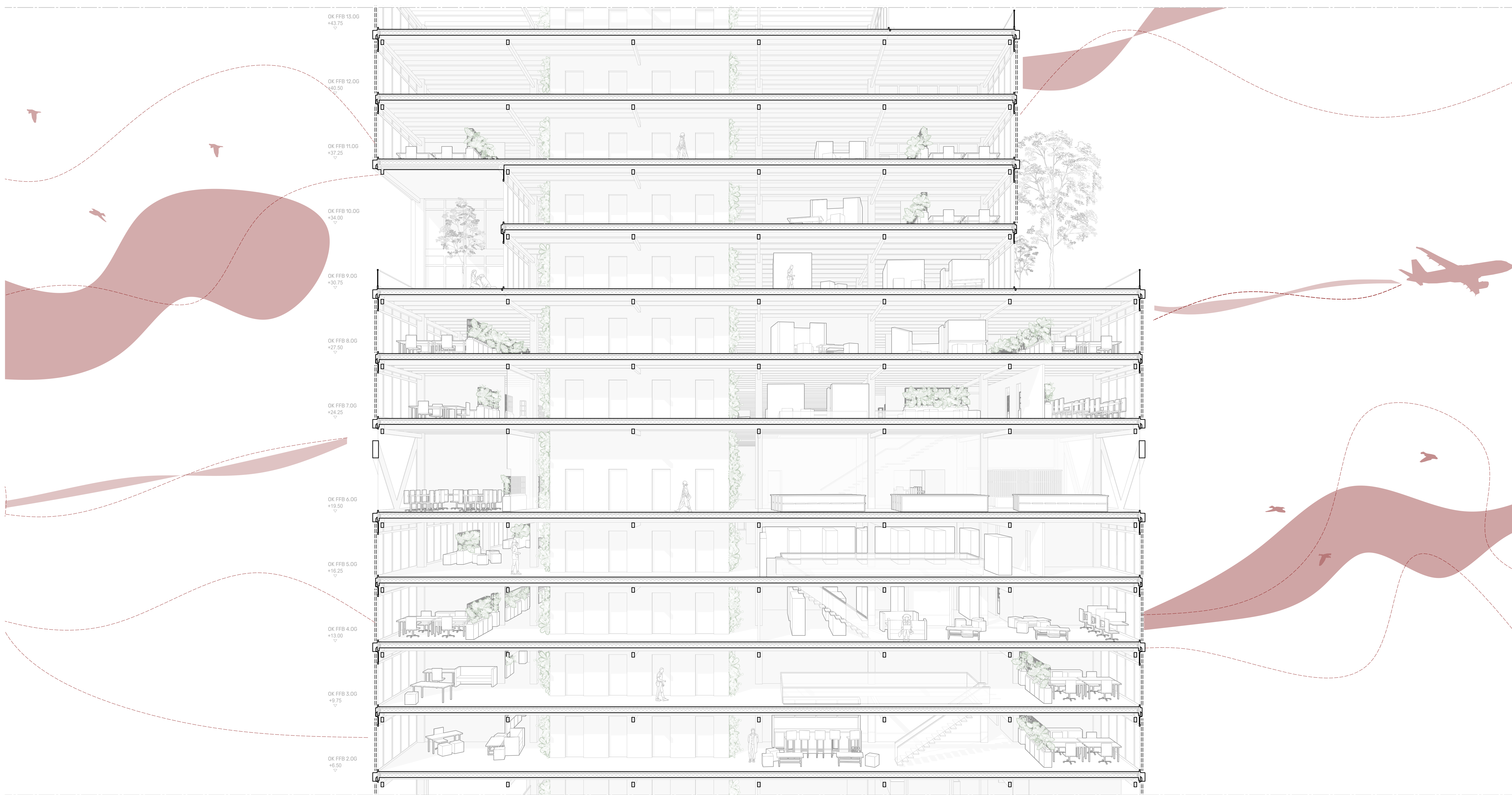
Schnittperspektive (Ausschnitt) | 2. bis 13. Obergeschoss M 1:100
