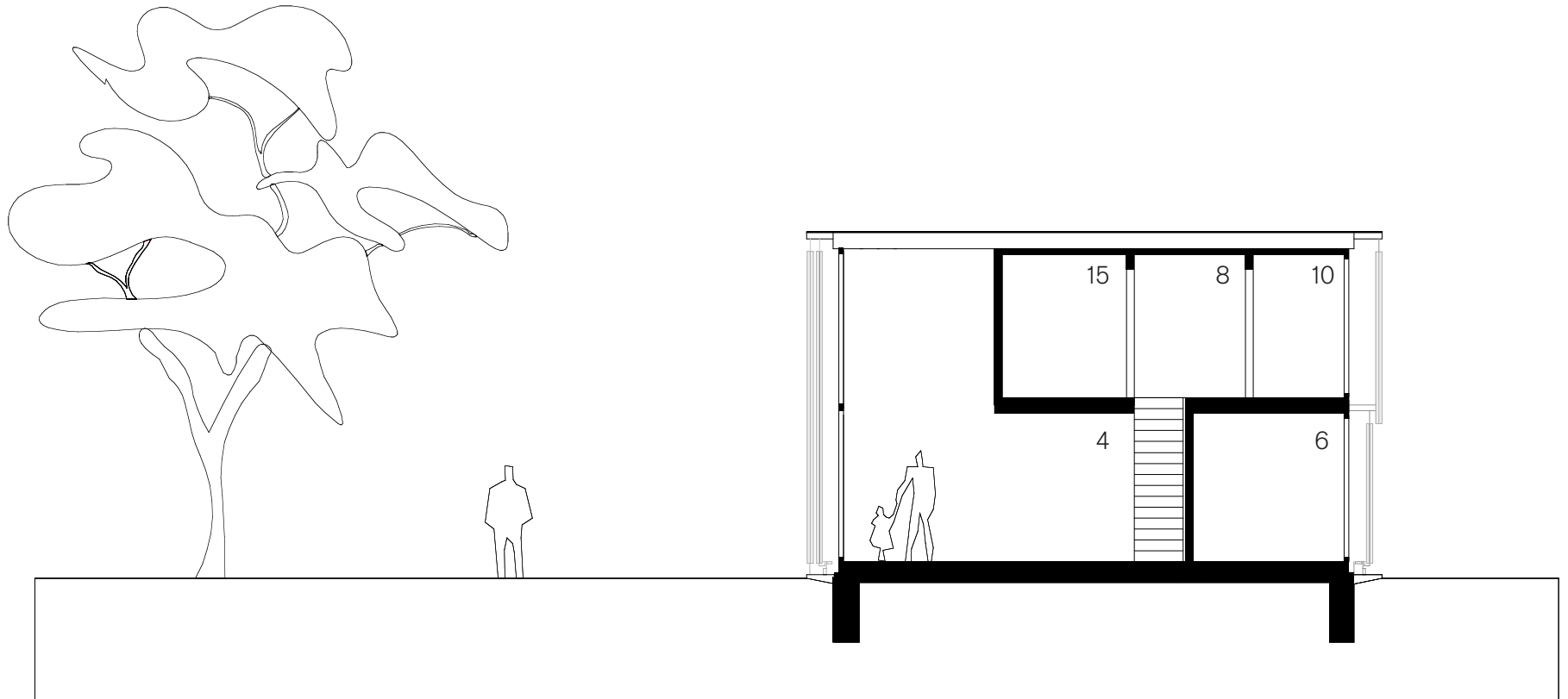
Schnitt M 1_100
