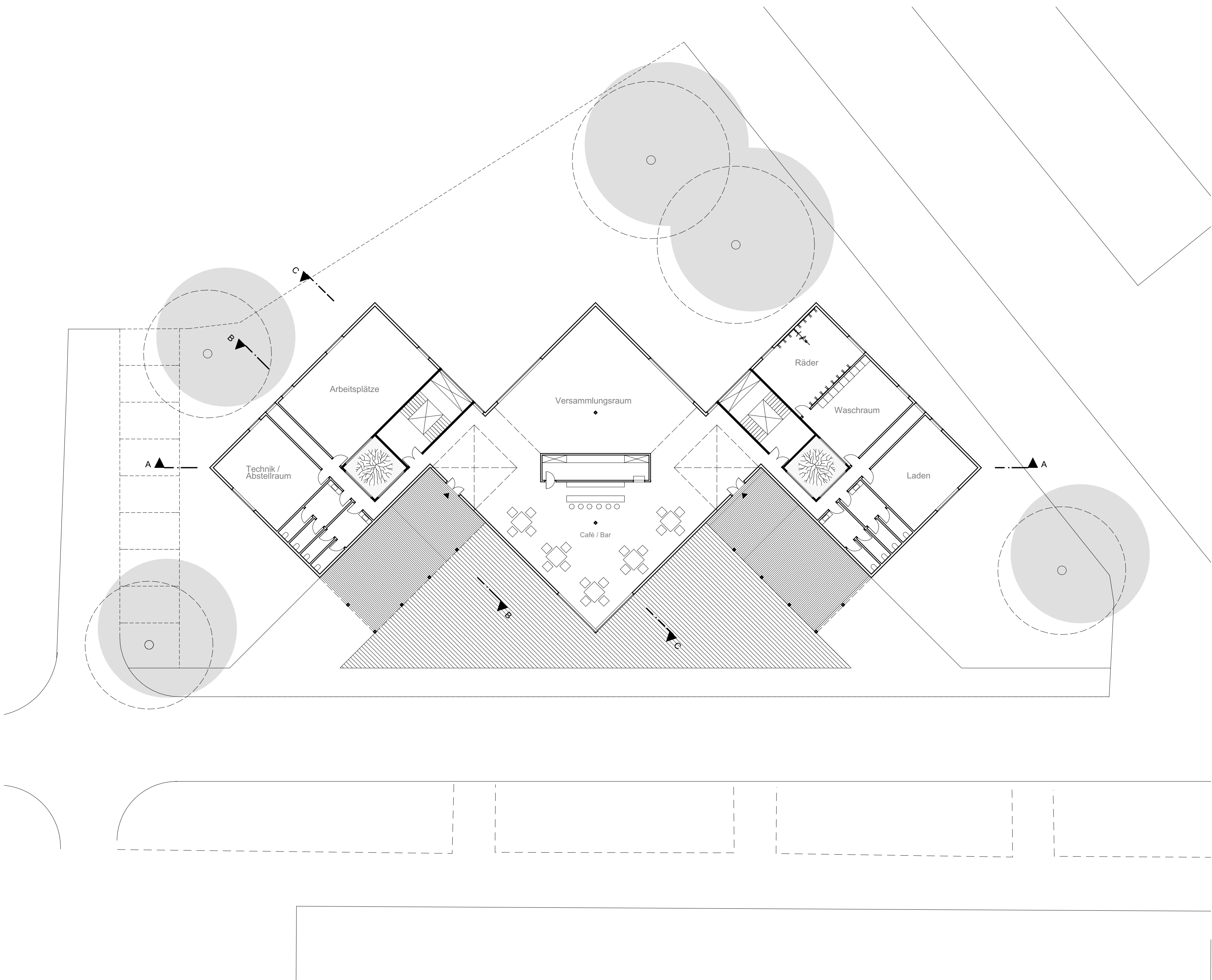
Grundriss EG
