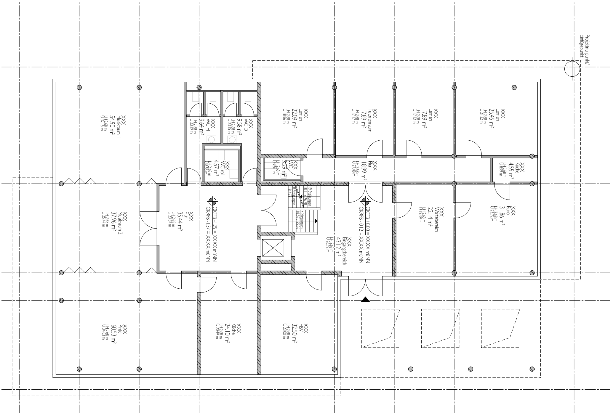
Grundriss Erdgeschoss
