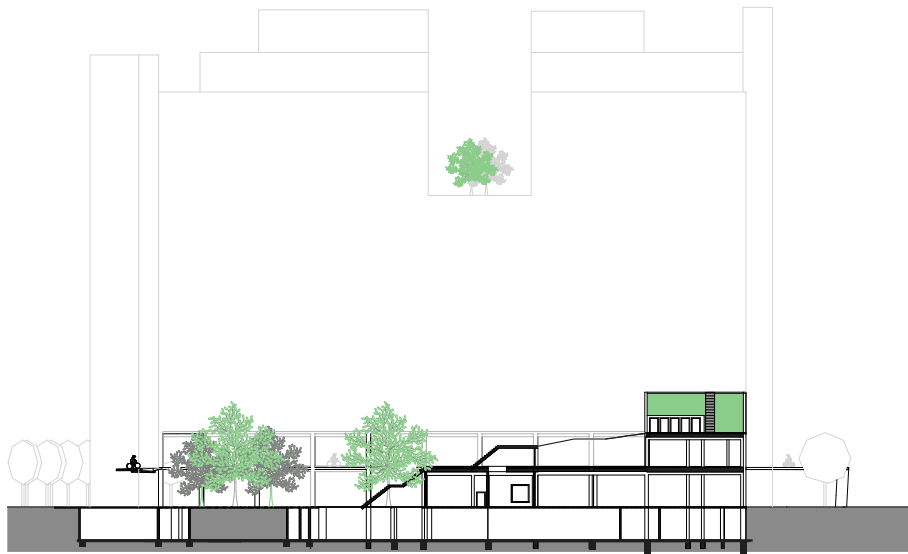
Ansicht Süd
