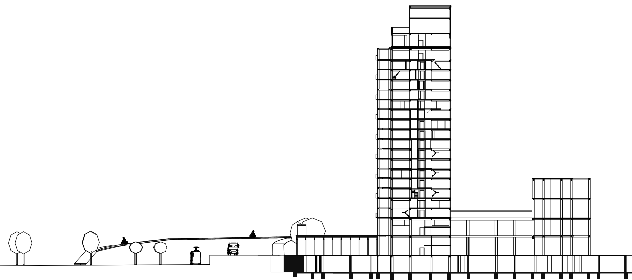
Schnitt B
