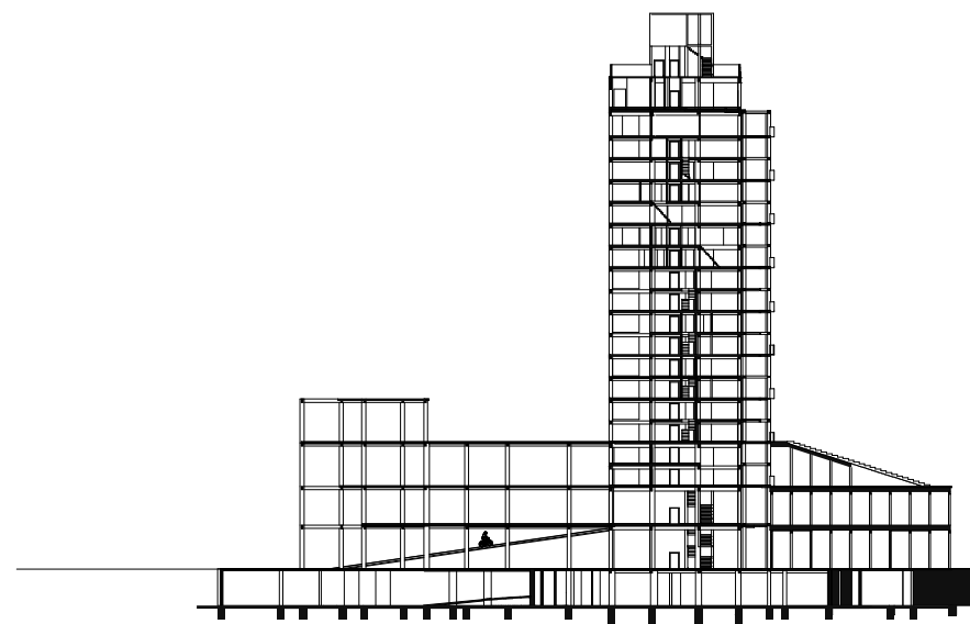
Schnitt C
