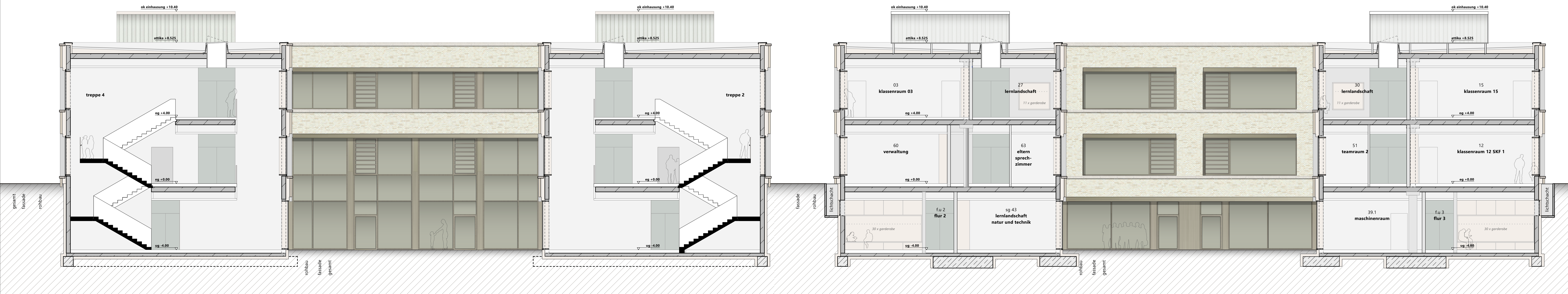
SCHNITT 3-3
