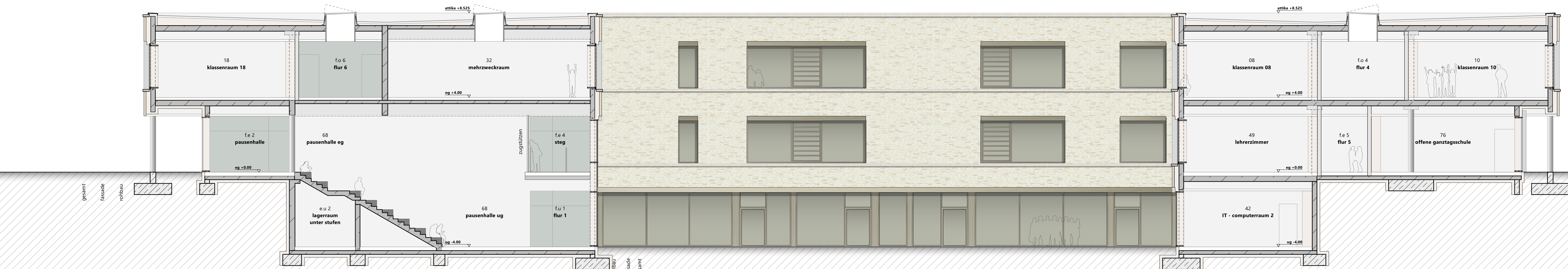
SCHNITT A-A
