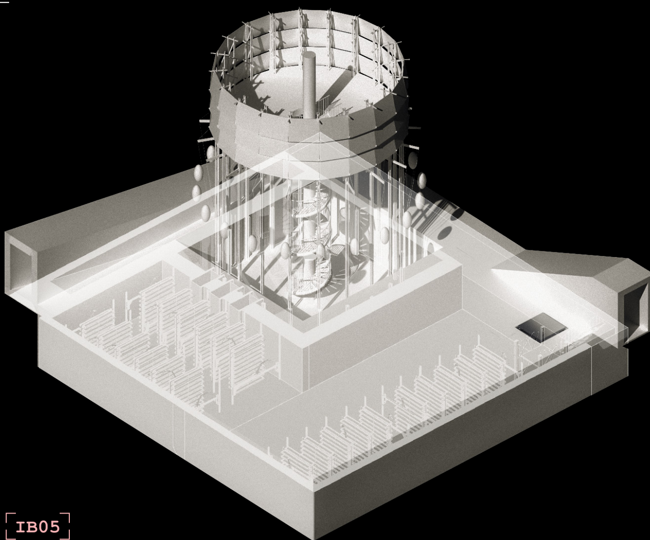
[ ISOMETRIE UG ]
