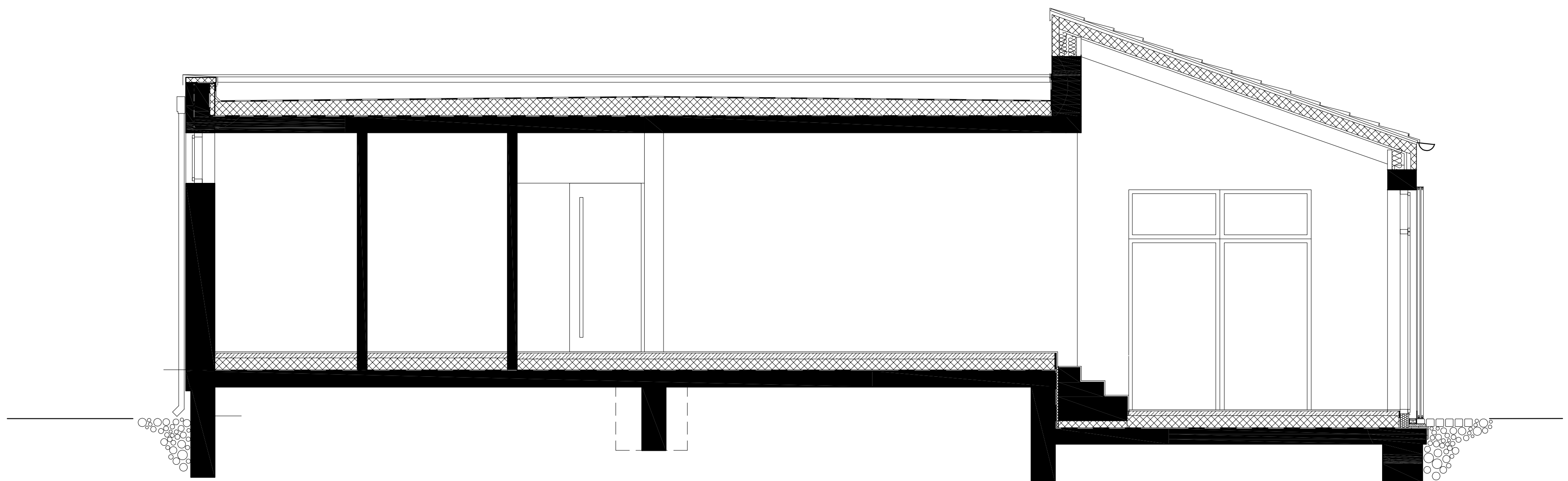
Schnitt AA
