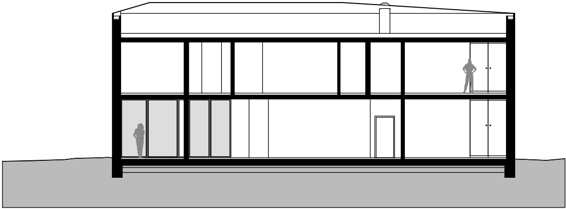
SCHNITT CC
