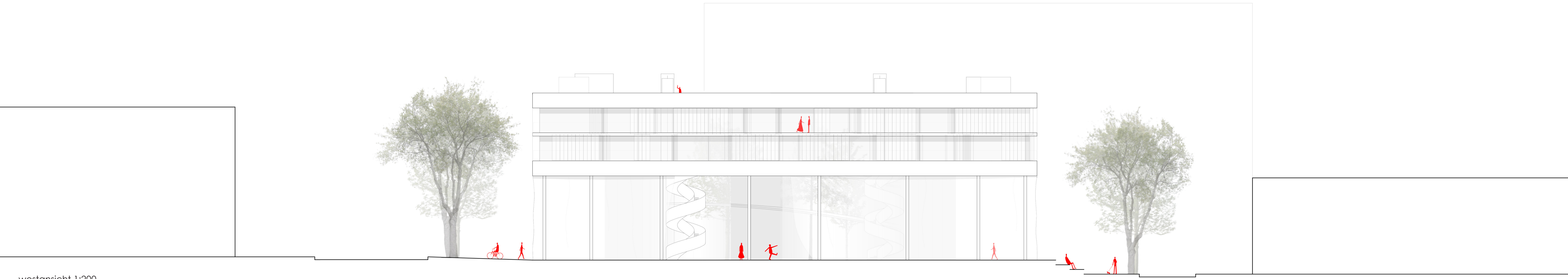
westansicht 1:200
