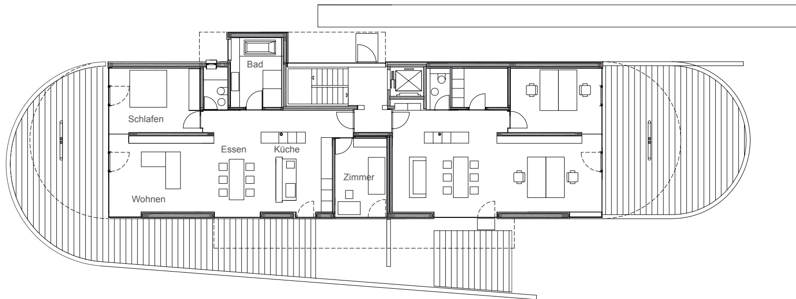
Grundriss EG
