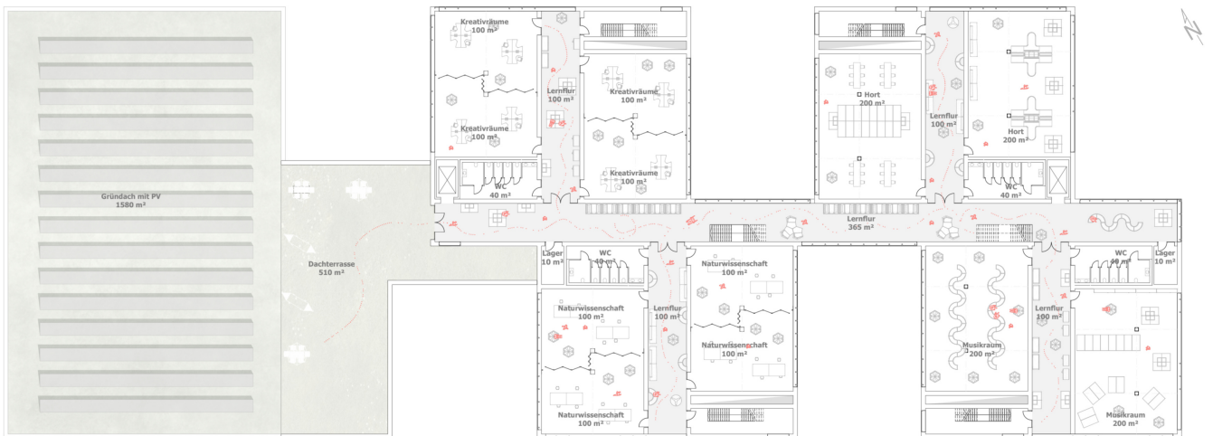
Grundriss 2. Obergeschoss M 1_200
