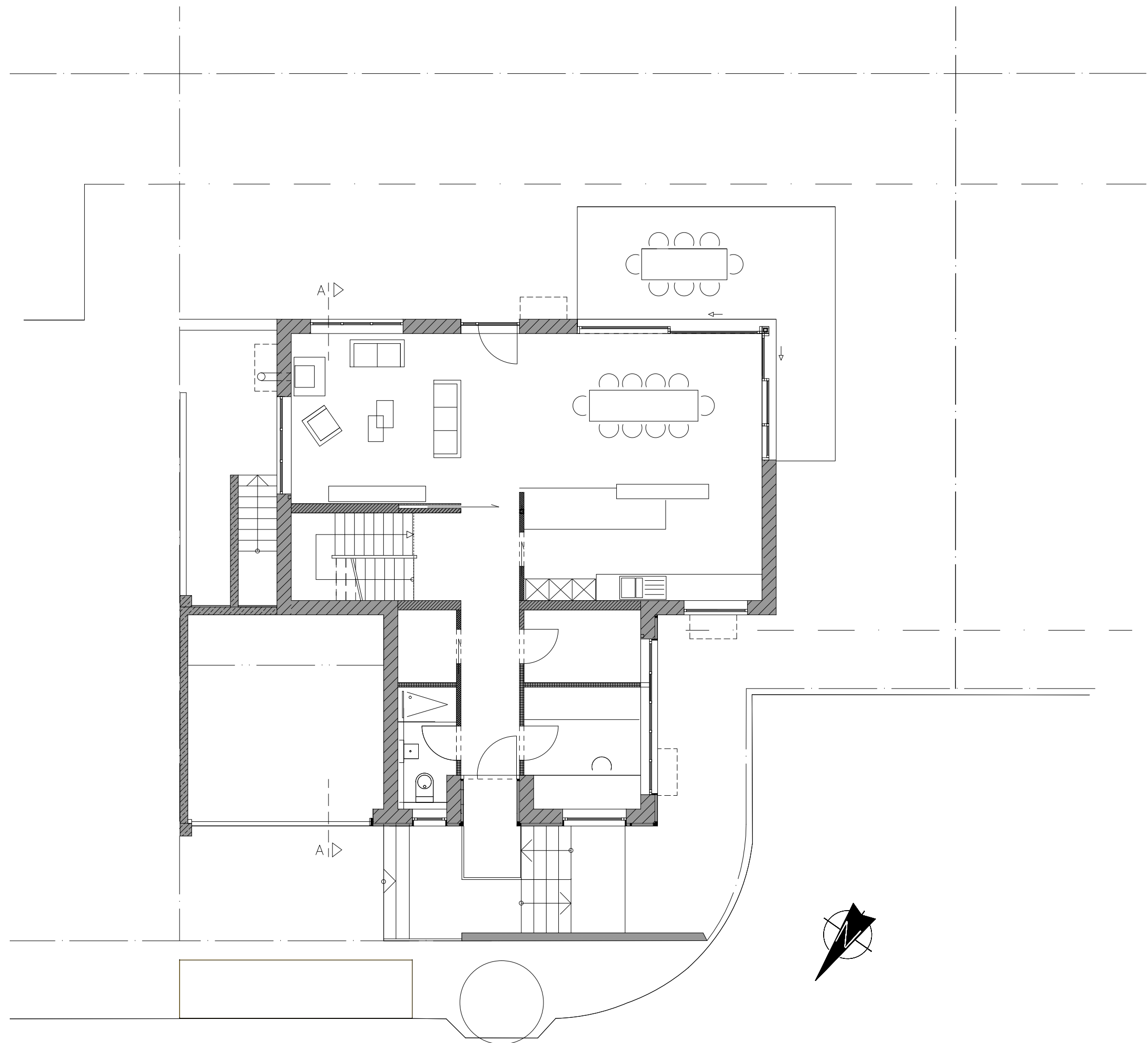
Grundriss EG
