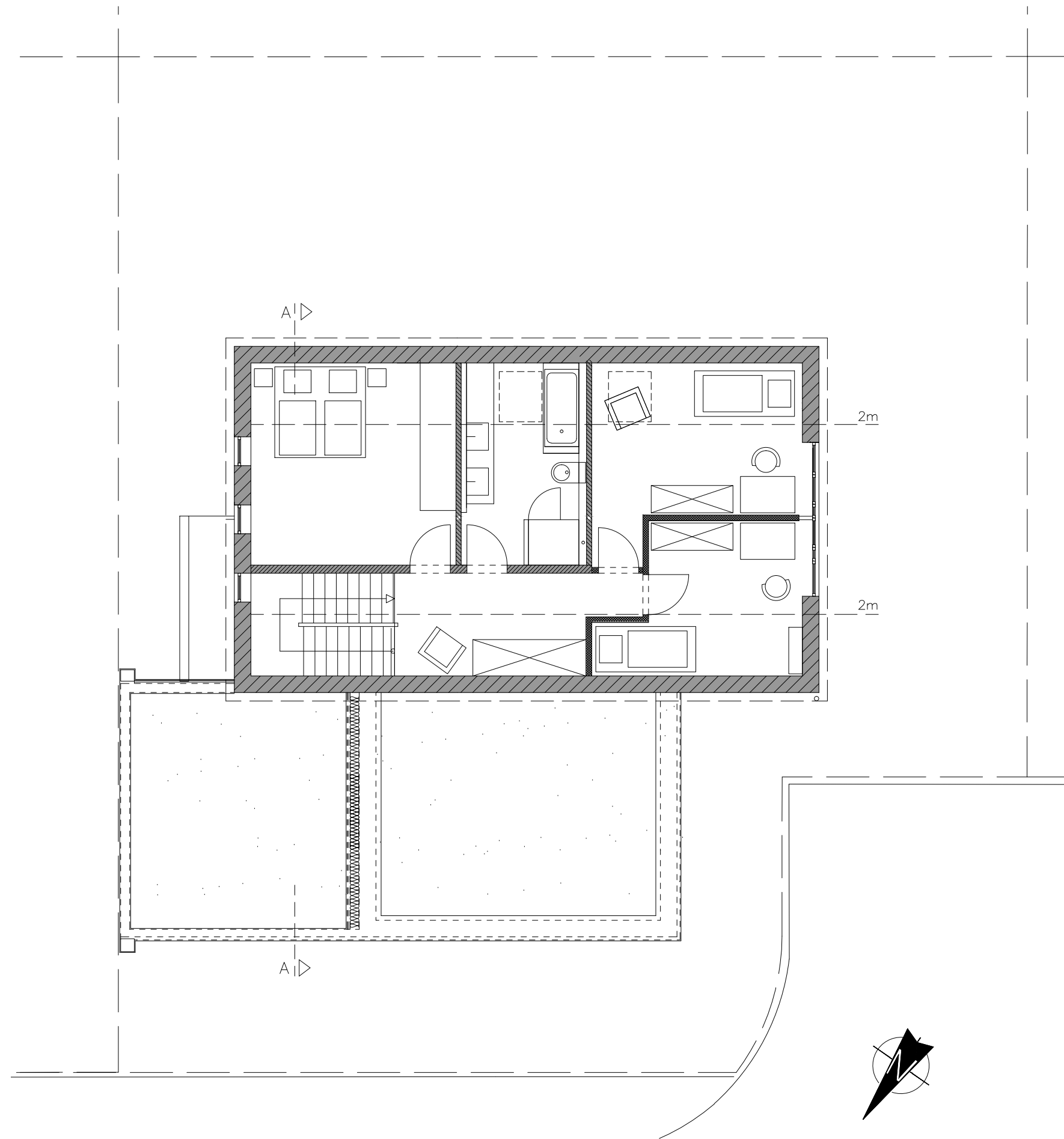
Grundriss OG
