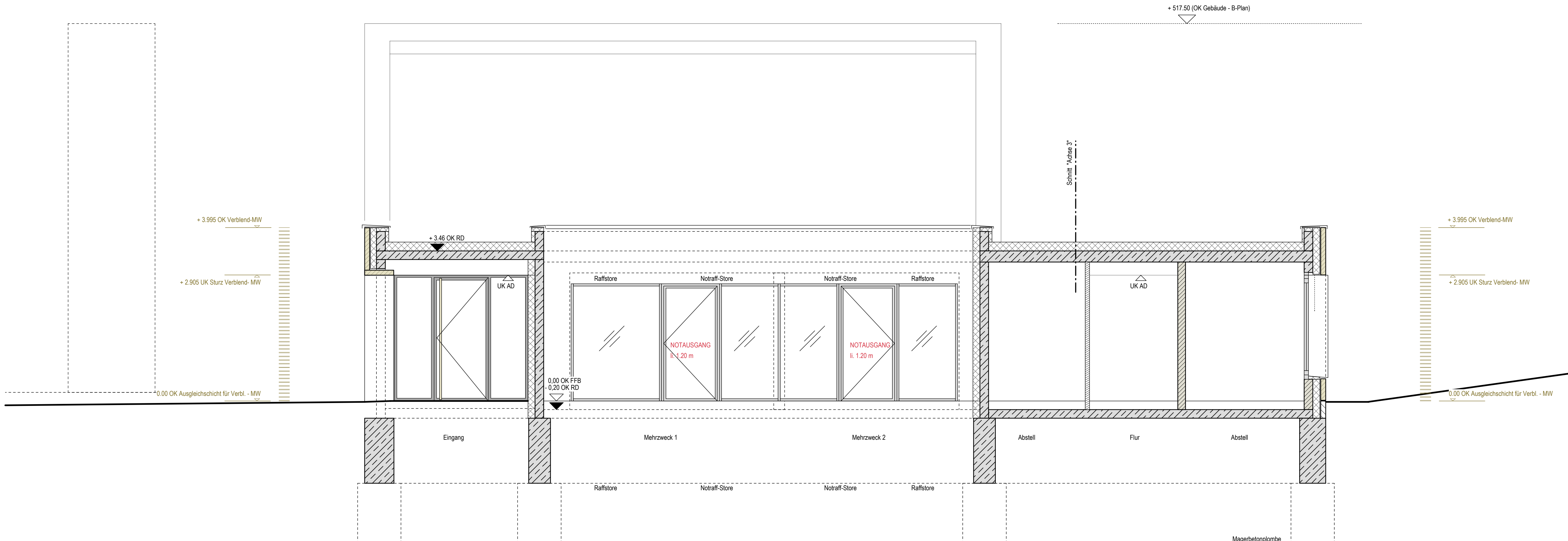
Schnitt B-B Maßstab 1 / 50
