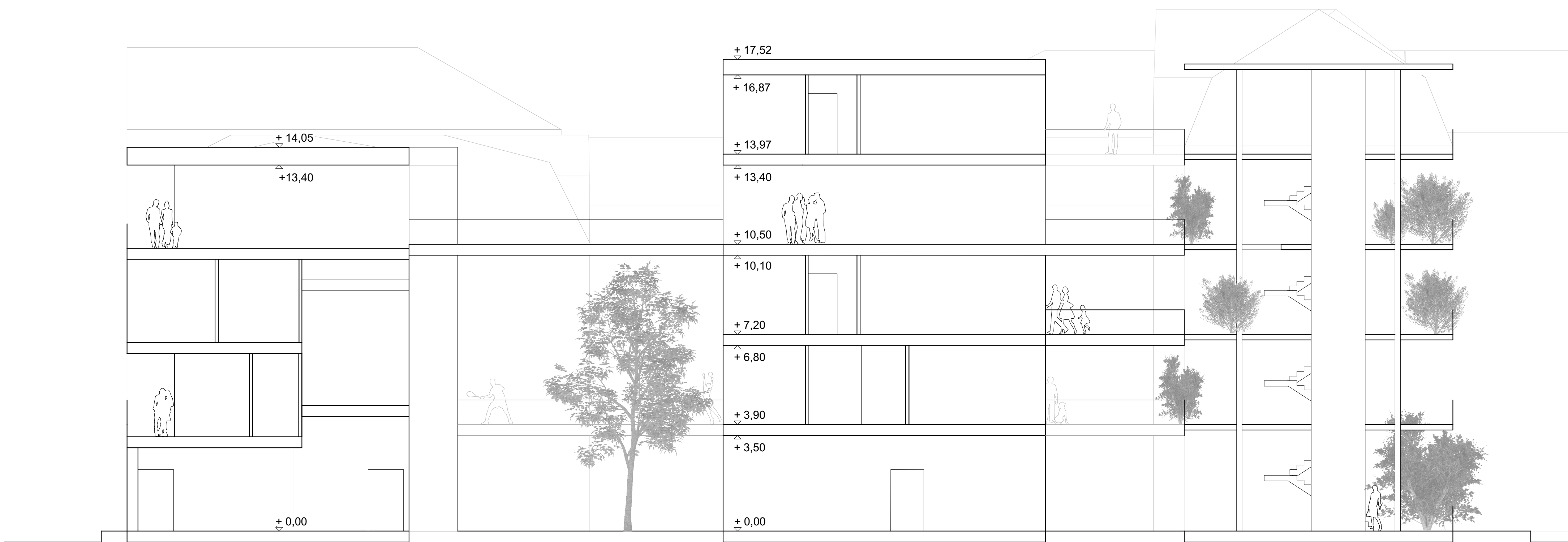
Schnitt C-C M 1:100
