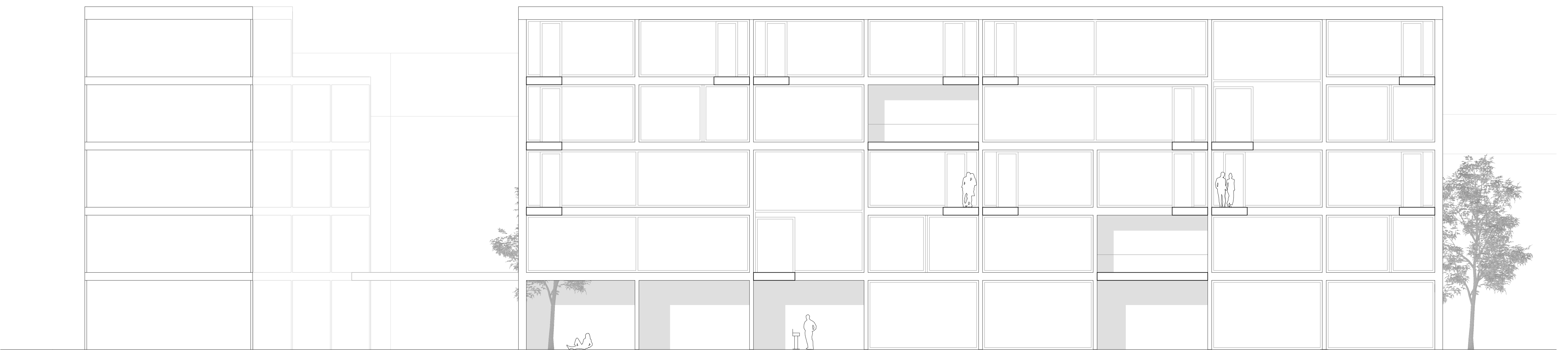
Schnitt D-D M 1:100
