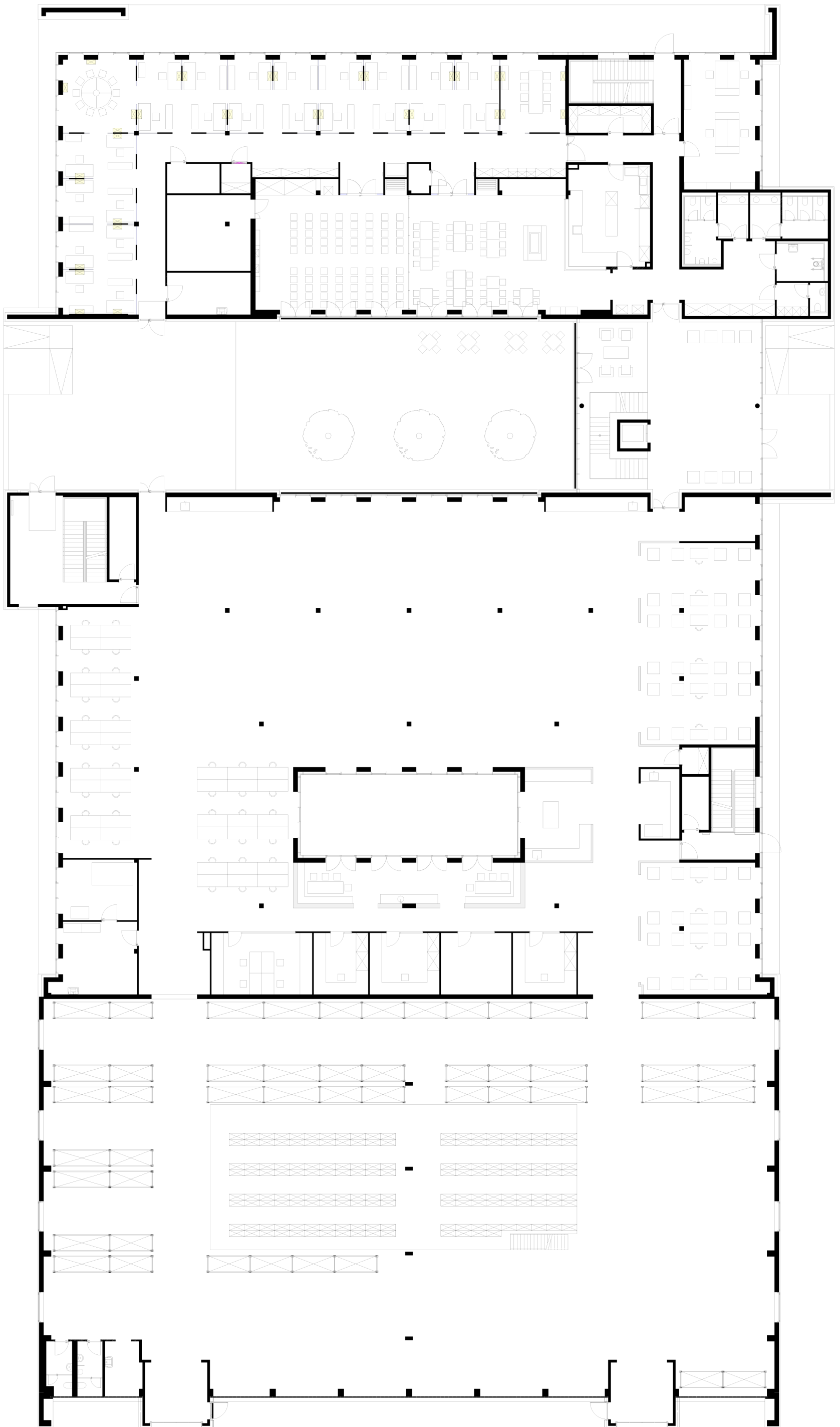
grundriss erdgeschoss - m 1:250
