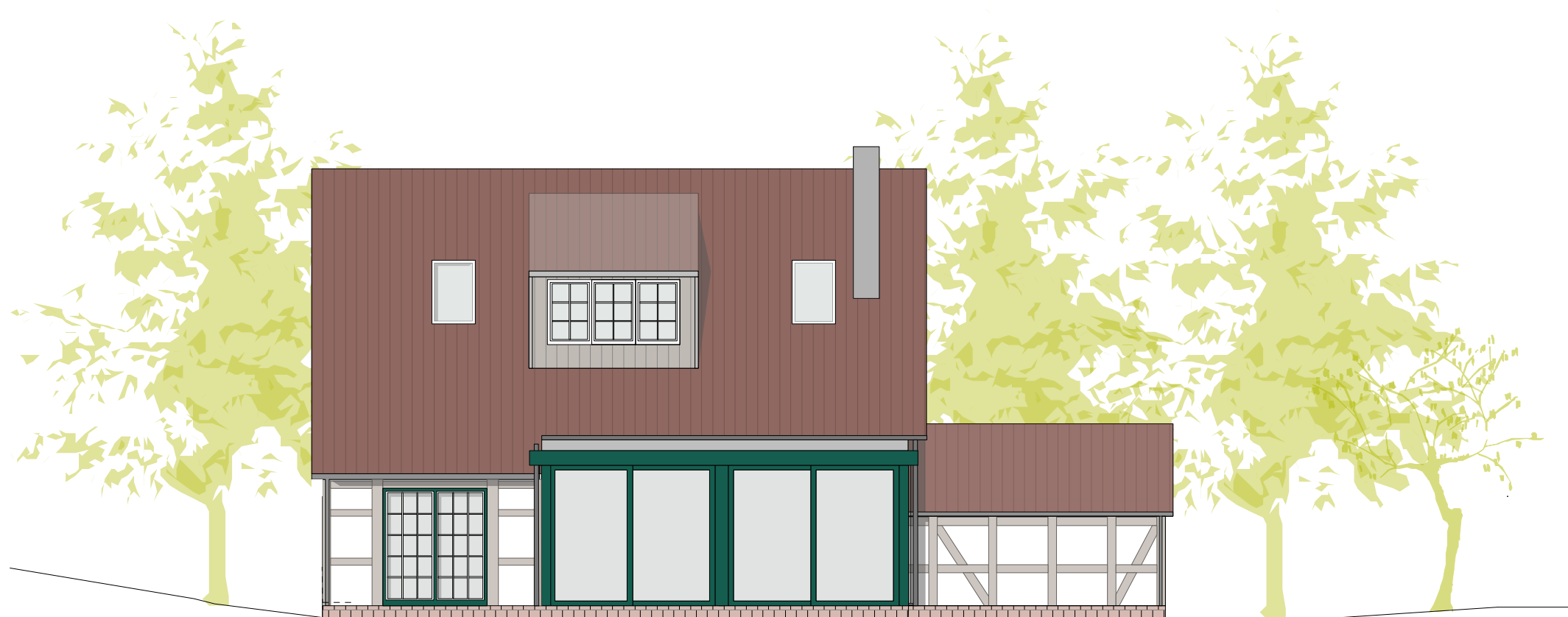
Ansicht West
