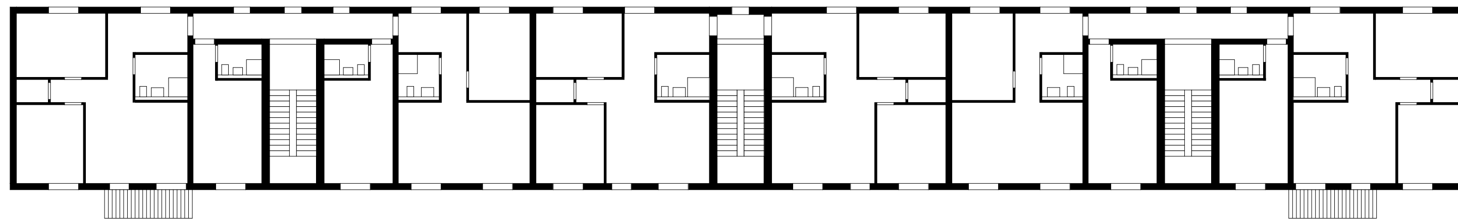
Platensiedlung, Frankfurt a. M. Regelgeschoss - Aufstockung 1 1:200
