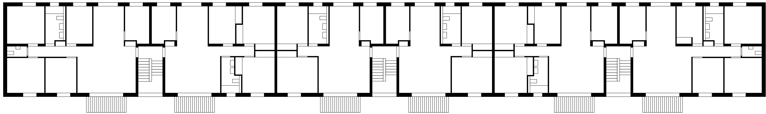
Platensiedlung, Frankfurt a. M. Erdgeschoss 1:200
