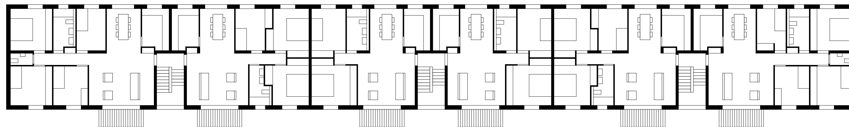
Platensiedlung, Frankfurt a. M. Erdgeschoss 1:200
