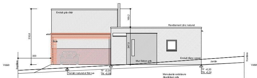
VUE RUE DU 17 FEVRIER
