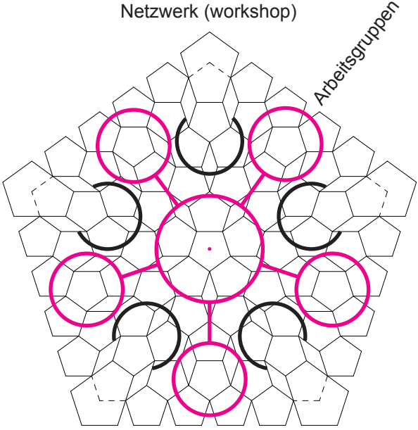
Netzwerk (workshop)
