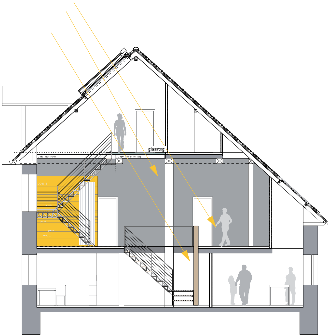
Schnitt b-b
