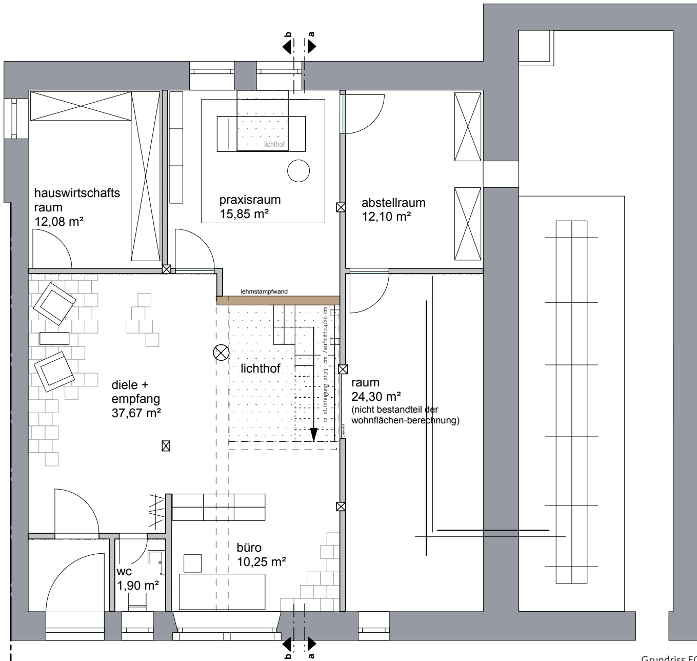
Grundriss EG
