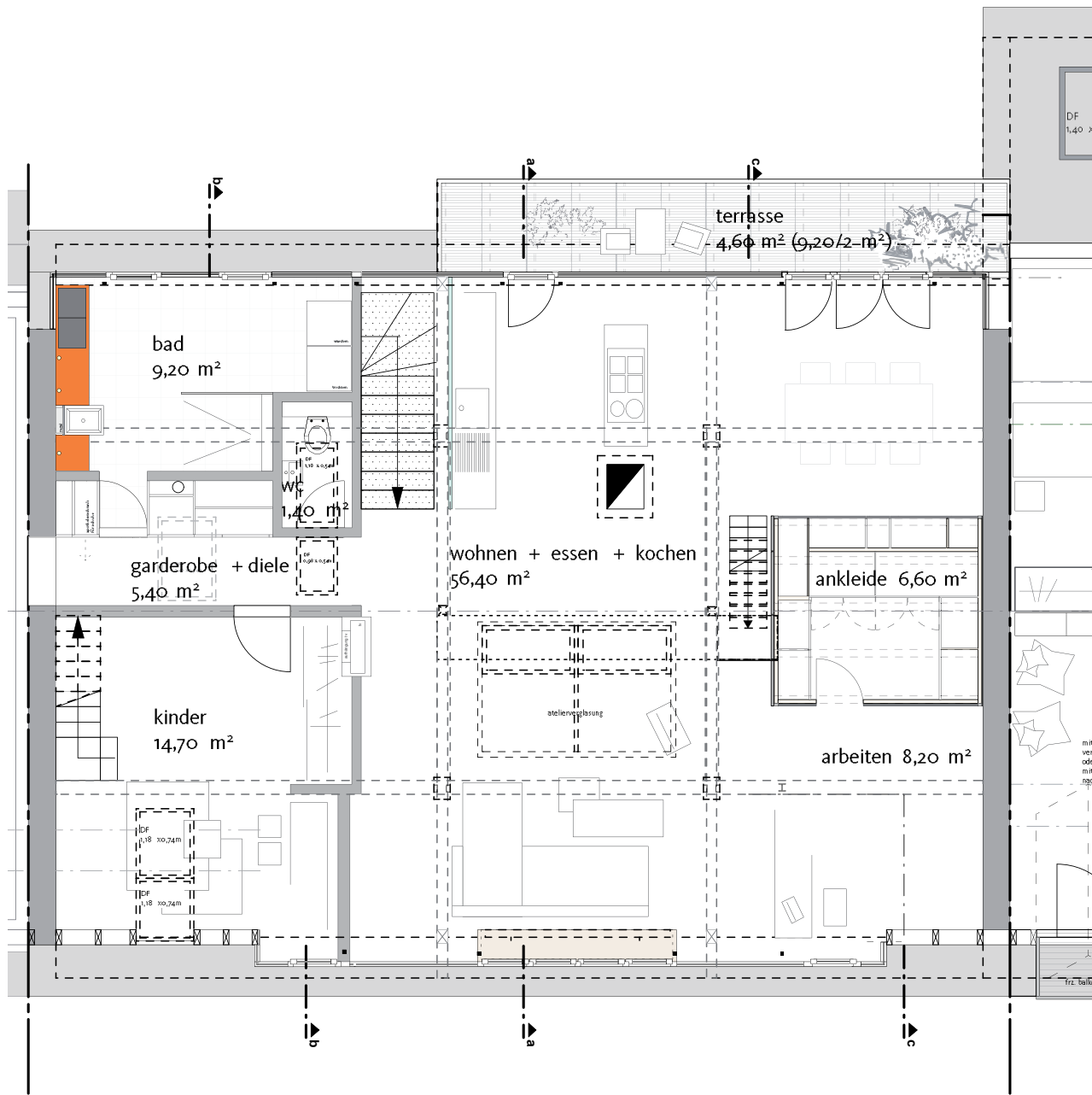
Grundriss Dachgeschoss
