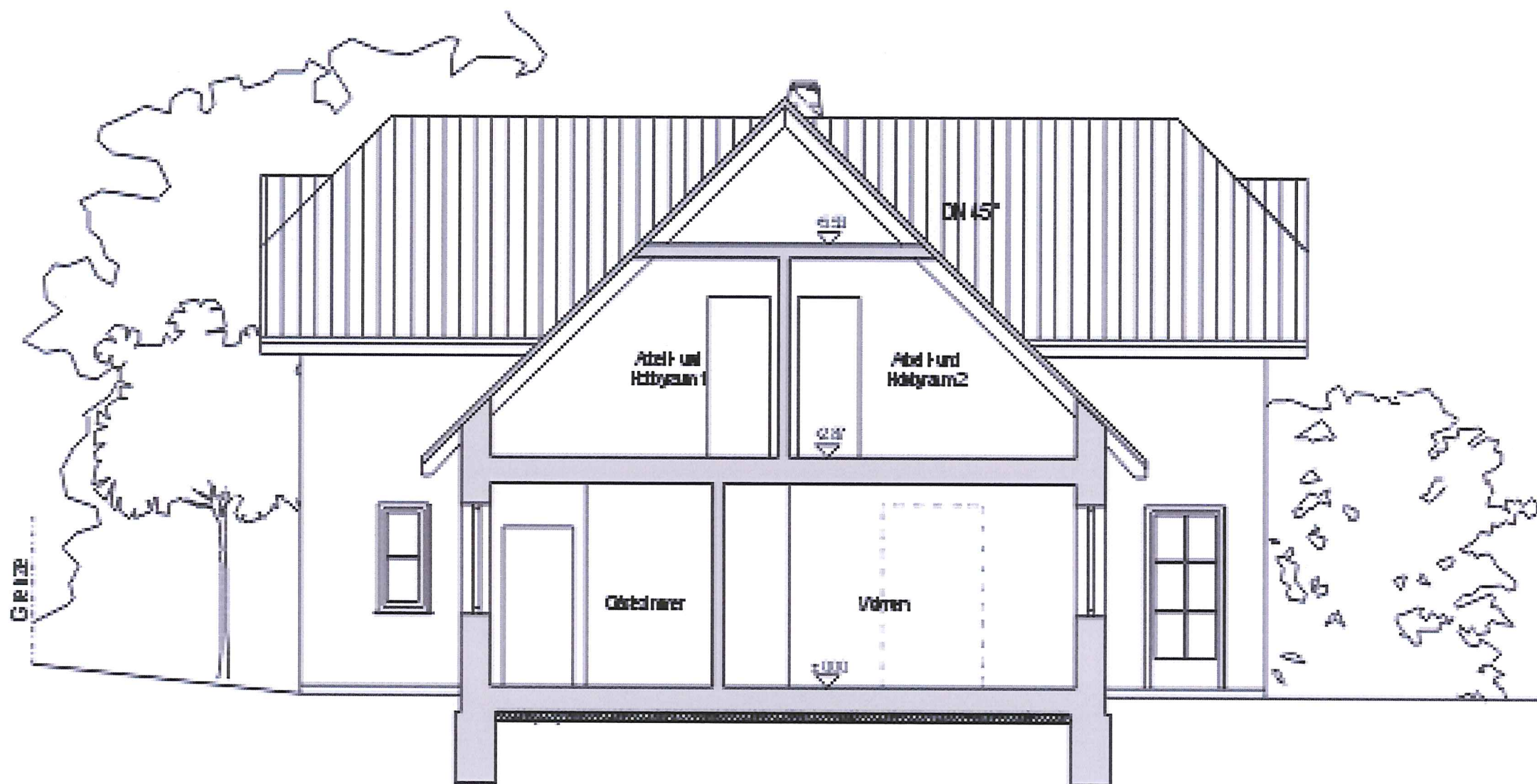
Schnitt A-A
