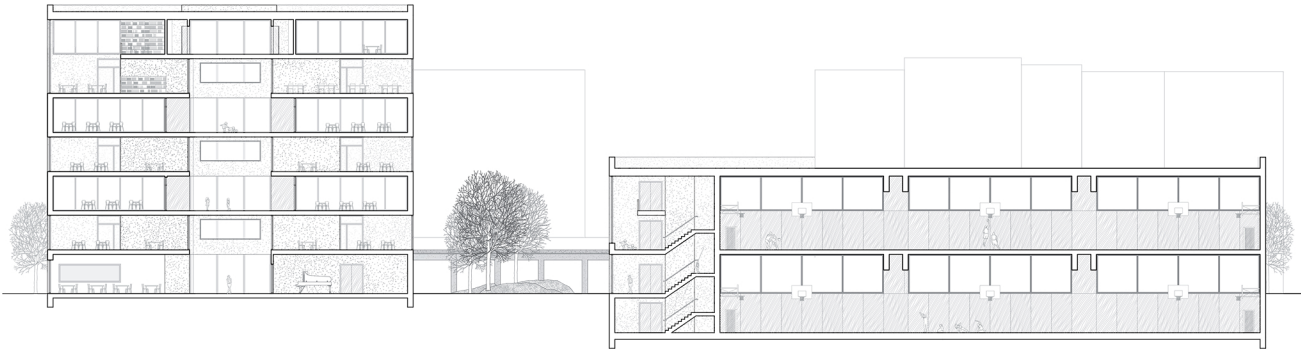
SCHNITT M 1_200
