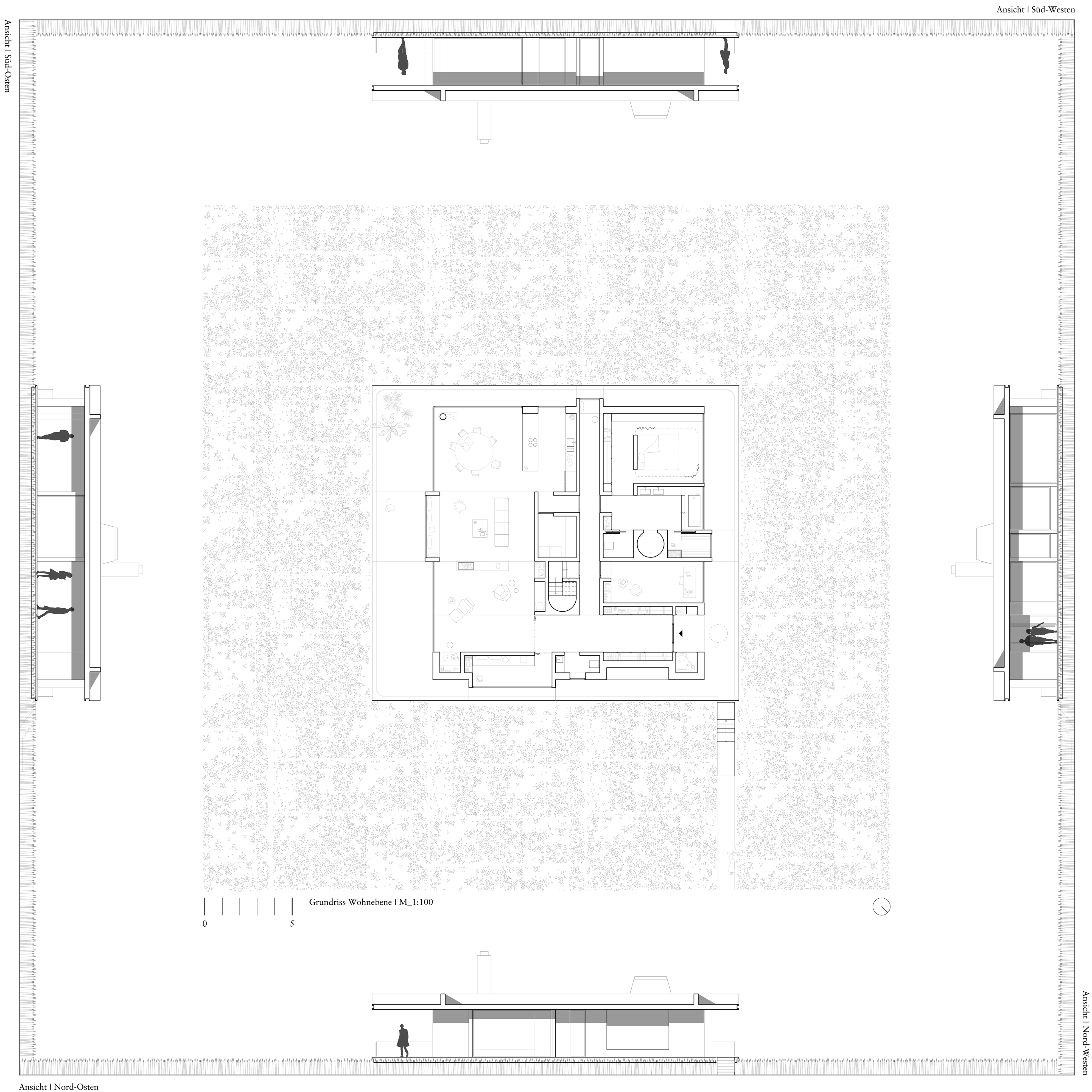
Ansicht | Nord-Osten
