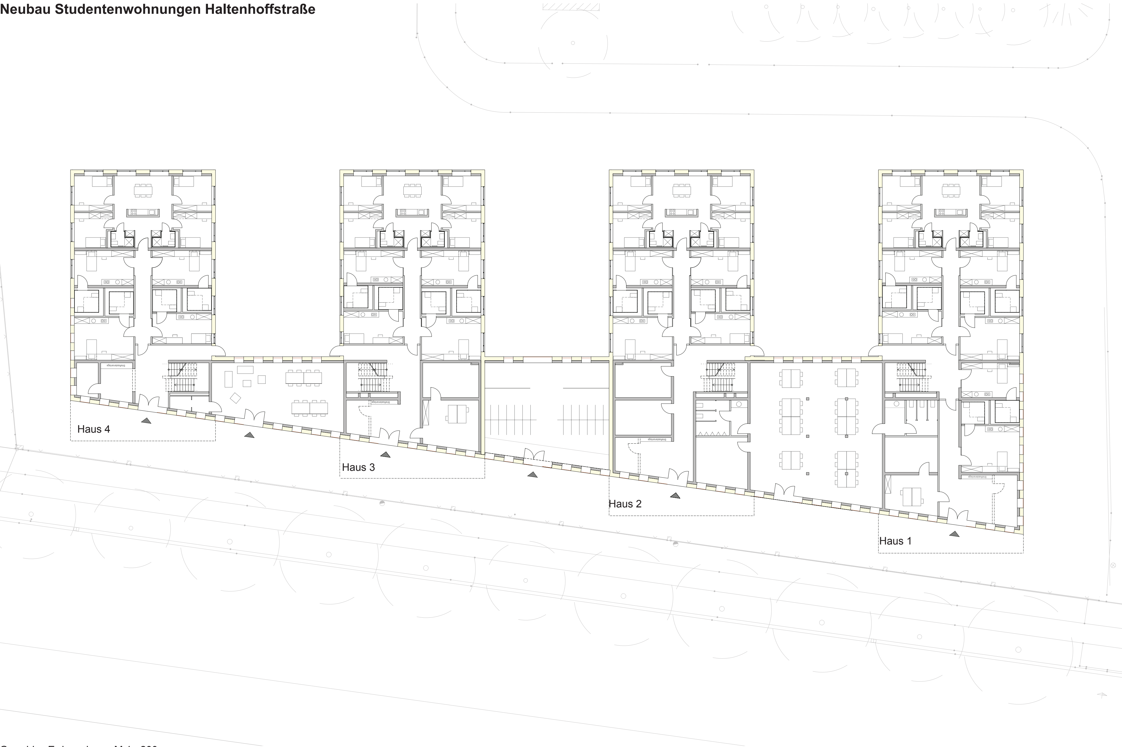
Grundriss Erdgeschoss, M 1 : 200
