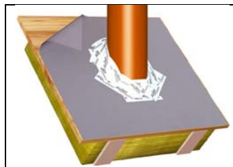
Abb. 7: Dunstrohr außen
