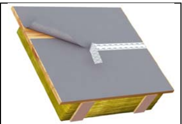
Abb. 6: Überlappung außen
