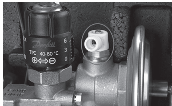
Entlüftung / Air valve
