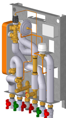
EvoFlat Reno mit Rohrleitung nach unten (Standard) EvoFlat Reno with piping downwards (Standard)
