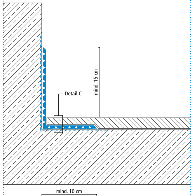
Wandanschluss mit Fremdbelag
