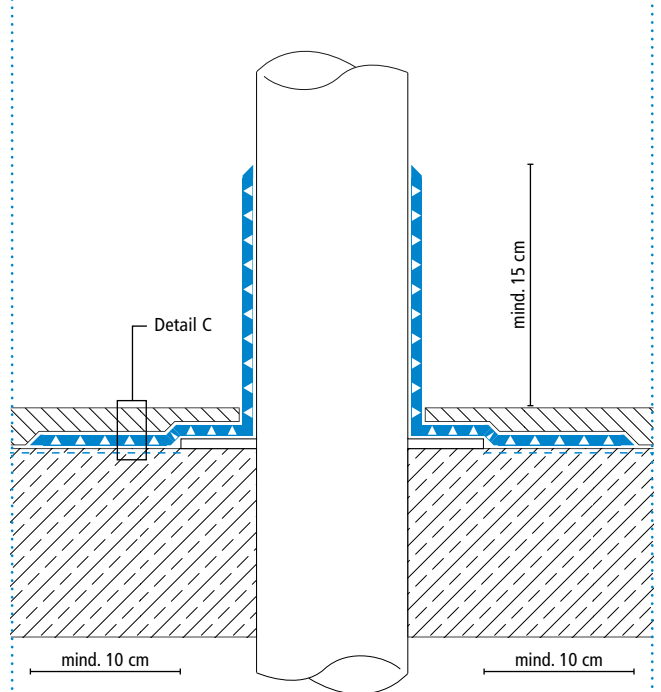
Durchdringung mit Fremdbelag
