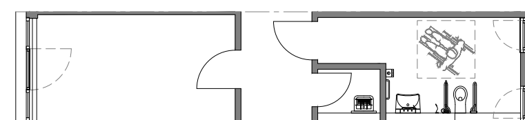
ML 3000 TO-B Sanitär-Modul mit behindertengerechtem WC
