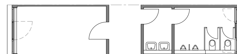
ML 3000 TO-H Sanitär-Modul mit WC (H)
