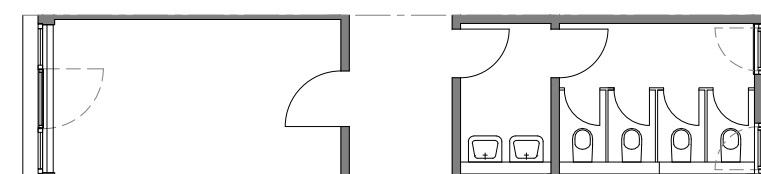
ML 3000 TO-D Sanitär-Modul mit WC (D)
