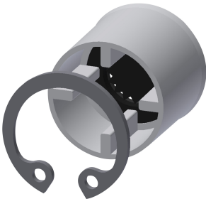
Durchflussmengenregler 0,20l/s
