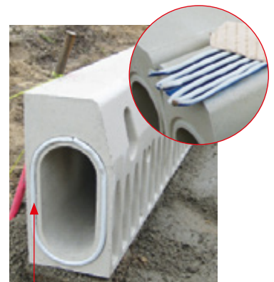
■ Dichtstoff in Nut
