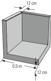
90°-Mauerscheiben-Außenecke, einteilig 12er SB, bis 1,55 m
