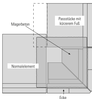
Ecke mit Passstück und Aufbeton
