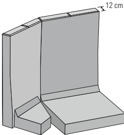
135°-Mauerscheiben-Außenecke, zweiteilig (aus Eck- und Normalelement) 12er SB, Sonder-MS
