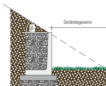
Der Einsatz der Winkelstützmauer sorgt für einen stabilen Zustand des Geländes.
