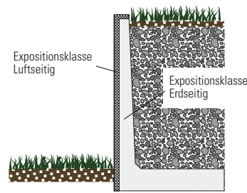
Lage der Expositionsklassen bei KANN Mauer-scheiben
