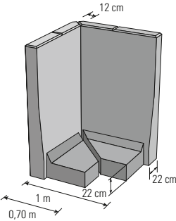
90°-Mauerscheiben-Außenecke, zweiteilig 12er SB, Sonder-MS ab 1,80 m
