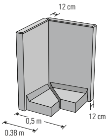
90°-Mauerscheiben-Außenecke, zweiteilig 12er SB, Sonder-MS bis 1,55 m
