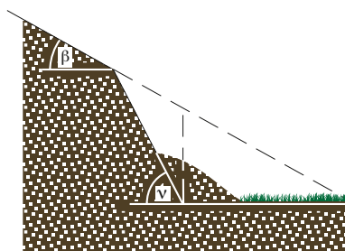
Senkrechte Abschtachtung: Das Gelände rutscht nach.
