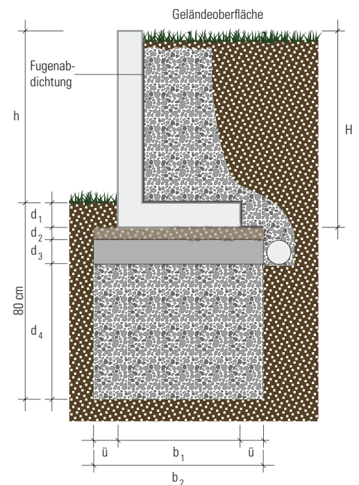
Aufbau der Fundamente Abmessungen s. Tab. links
