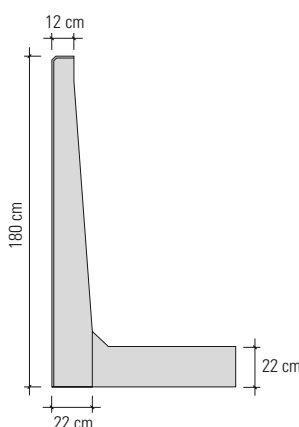
MS ab 1,80 m mit schräger Rückseite
